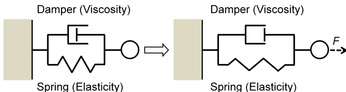
図 11 粘弾性体モデル (Kelvin-Voigt model)
