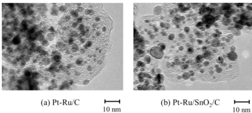
Fig. 5.3 STEM images of (a) PtRu/C and (b) PtRu/SnO 2 /C.
