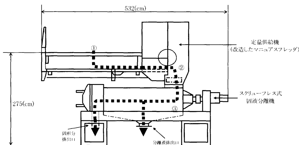
図1 セミソリッドふん尿用固液分離装置の概要
