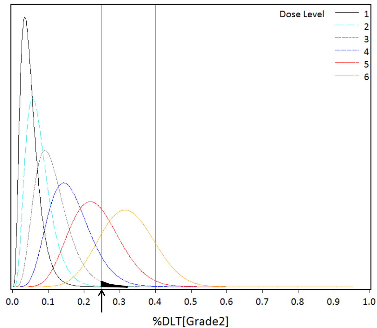
Posterior distribution
