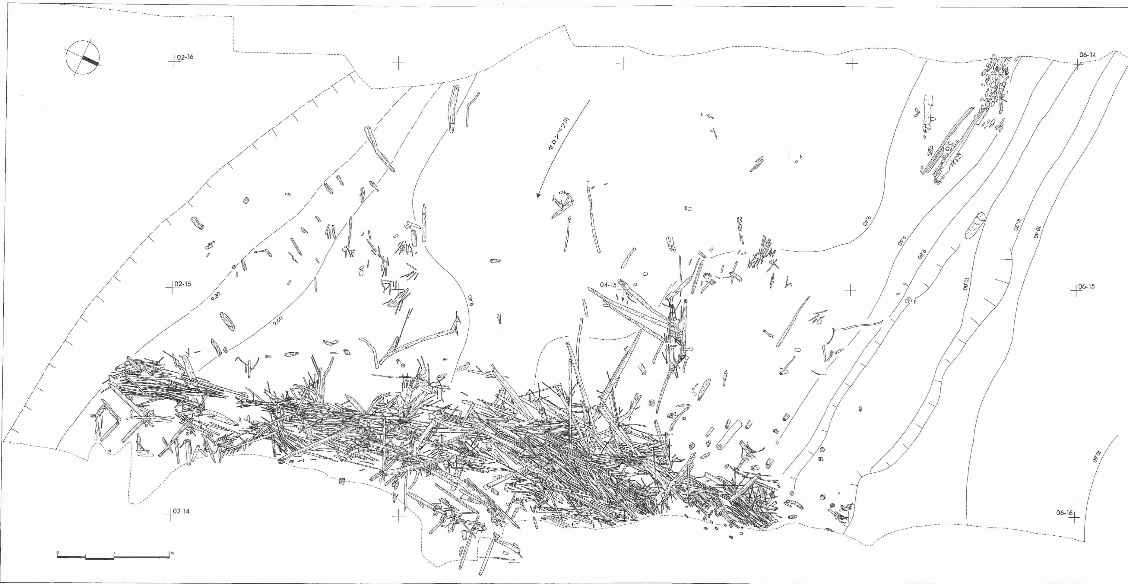
第7図 堰状遺構(テシ)実測図
