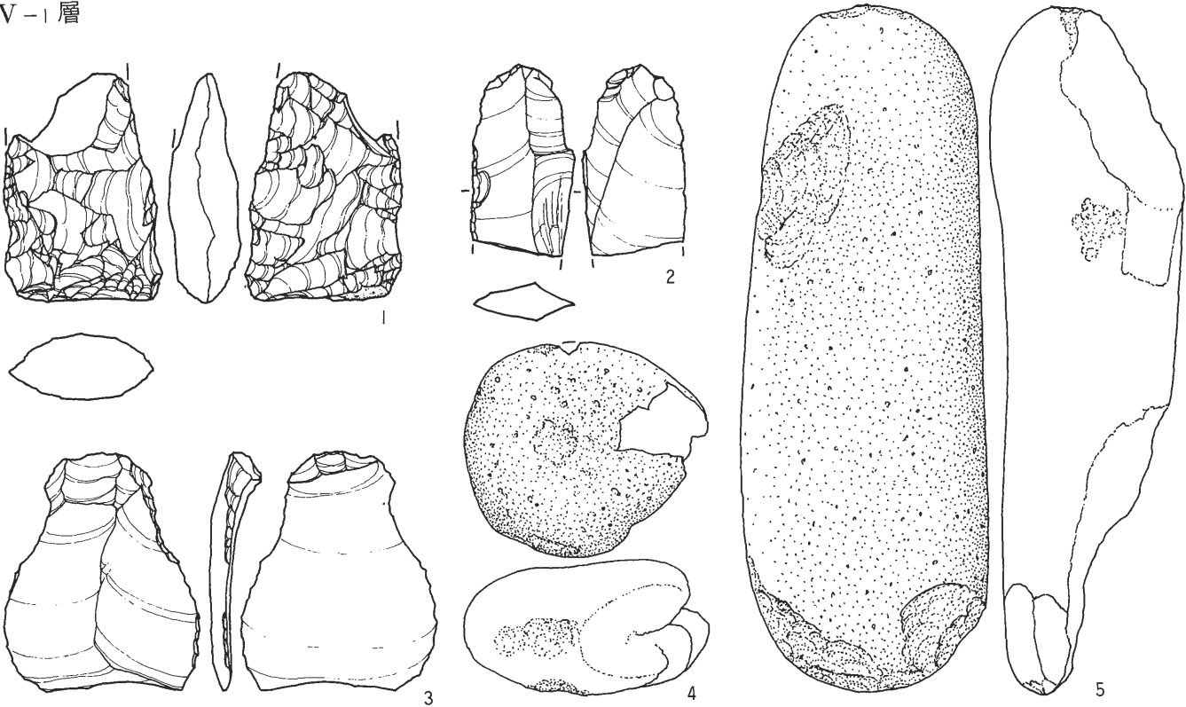
图9 中央道路共同溝（第4工区）地点出土石器(Ⅰ) (1~3, 6~9: 1/1, 4, 5, 10~12: 1/2)
