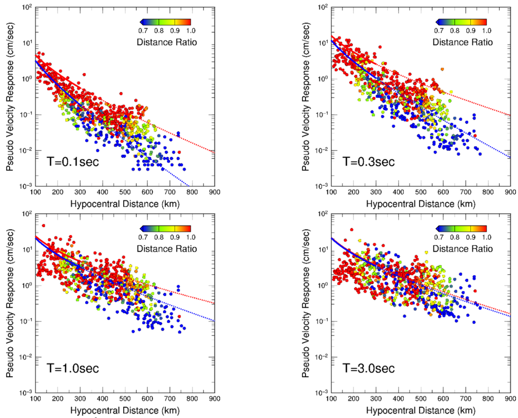
図9 No.7地震（プレート境界地震: M_W 7.3 ）による擬似速度応答値（観測）の距離減衰特性（赤・青線はDhakal式による予測値）
