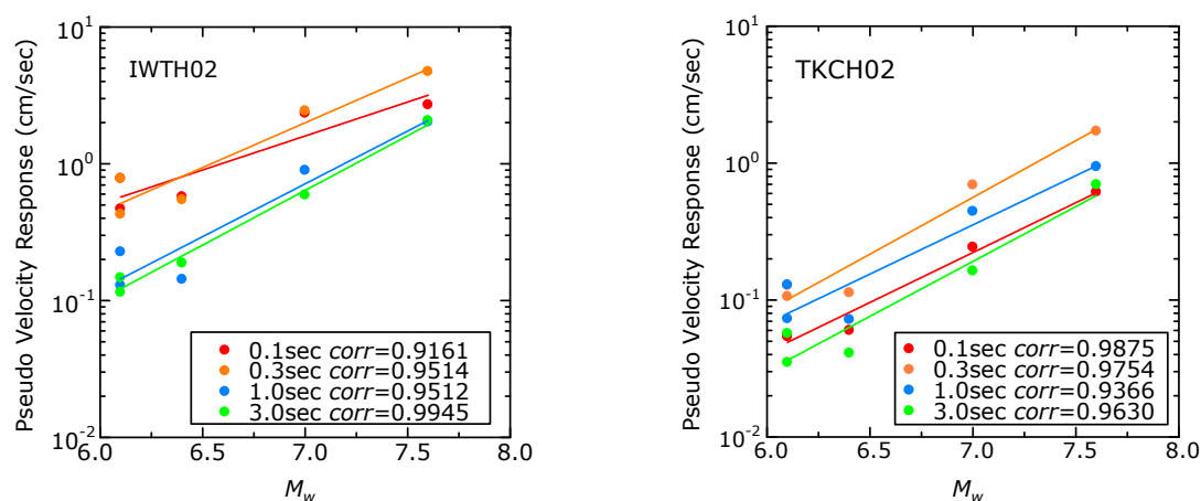
図13 2観測点における5地震の M_W と擬似速度応答値の関係（実線は回帰直線であり、色が固有周期に対応している。）
