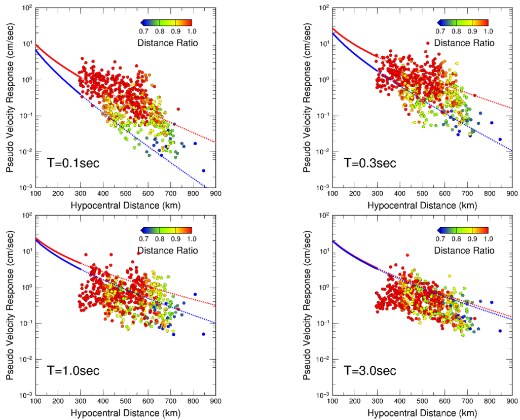
図10 No.1地震（アウターライズ地震: M_W 7.0 ）による擬似速度応答値（観測）の距離減衰特性（赤・青線はDhakal式による予測値）
