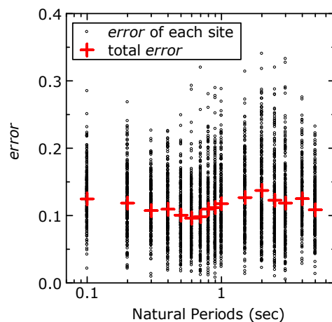
図17 観測値とSS-GMPEによる予測値の誤差（標準偏差）
