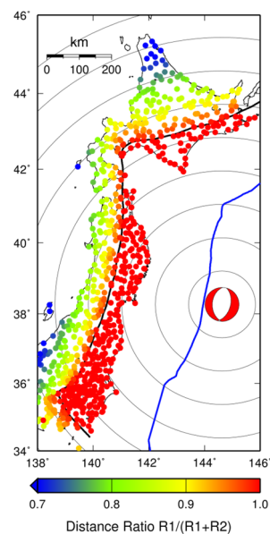
図5 No.2地震のDistance Ratioの空間分布 (黒線: 火山フロント、青線: 海溝、 震央からの同心円は100km間隔)
