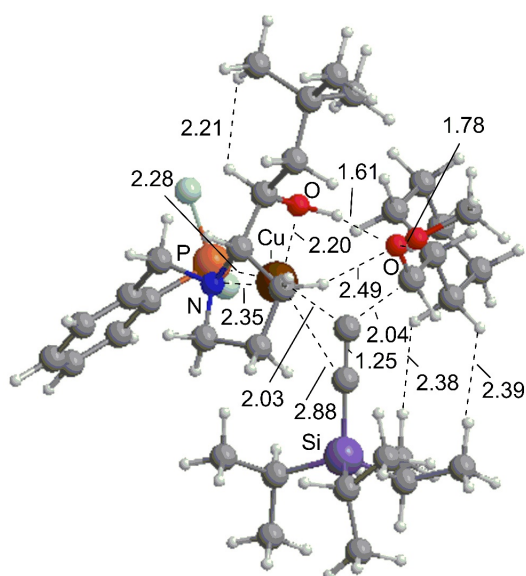
B-E6 2b-2-2-3-3-MeOH M
