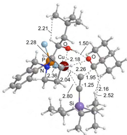
B-E6 2b-2-3-3 M
