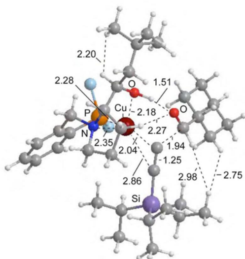
B-E6 2b-2-2-3 M
