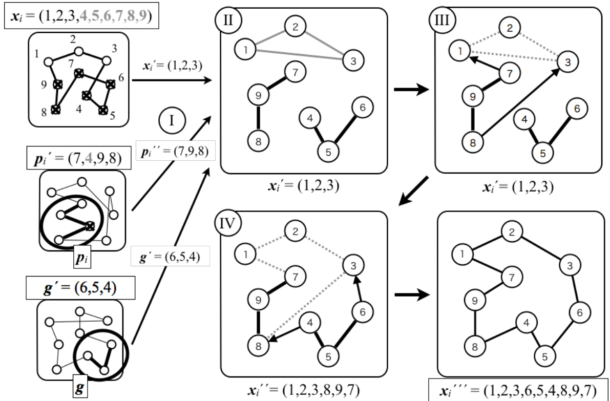
図 4.3 部分経路挿入の例
