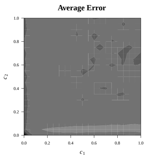
図 4.9 kroA200 に対し IPSO を 60000 ステップ適用し得られた解の平均誤差 \bar{e}_x .
