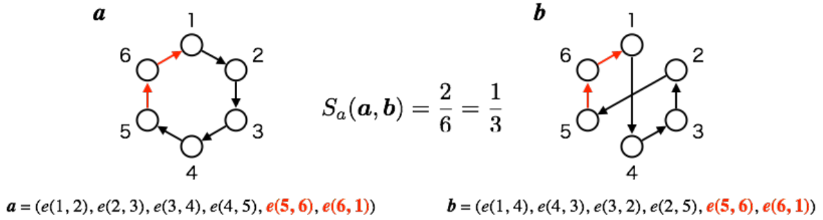
図 4.1 非対称 TSP における巡回路 a , b の類似度 S_a(a, b) . 非対称 TSP においては移動方向も意味があるため、向きも一致する辺のみ対象となる。
