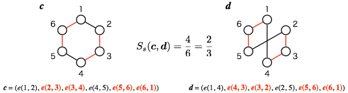
図 4.2 対称 TSP における巡回路 c , d の類似度 S_s(c, d) . 対称 TSP では辺の向きは関係ない。向きの一致している辺に加え、逆向きの辺も対象となる。
