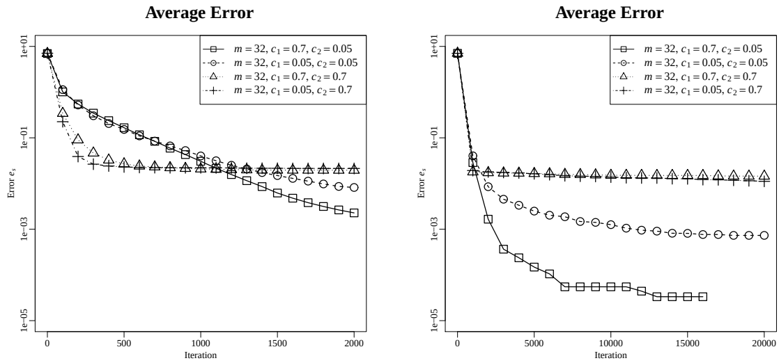
図 4.13 kroA100 に対し IPSO を適用し得られた解の平均誤差 e_x . 左図は 2000 ステップまで. 右図は 20000 ステップまで.
