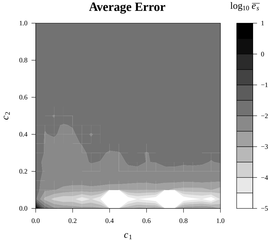
図 4.8 kroA100 に対し IPSO を 20000 ステップ適用し得られた解の平均誤差 \bar{e}_s .
