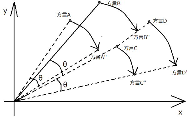
図 8. 原点を中心にある角度 \theta 回転させても方言 ABCD 間の相対的な関係が変わらないが X 軸 Y 軸の値が変わる.
