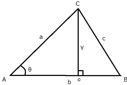
図 5. 三角形 ABC について. その 1
