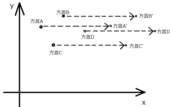
図7. あらゆる方向に方言 ABCD 間の相対的な関係を保ったまま，平行移動が可能であるがX軸Y軸の値が変わる．
