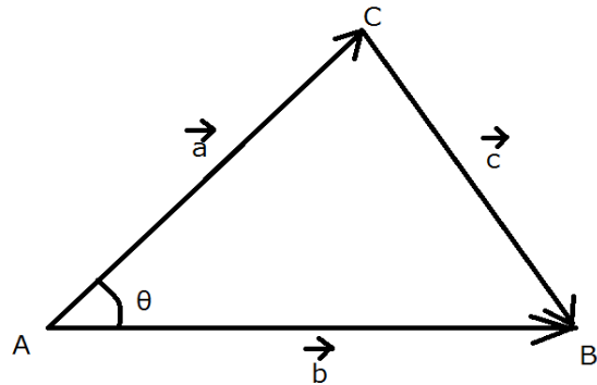
図 6. 三角形 ABC について. その 2
