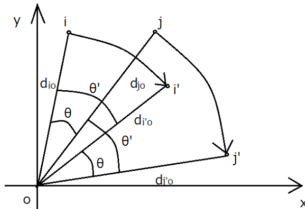
図 9. 各方言の座標の「重心」を原点に置いた図
