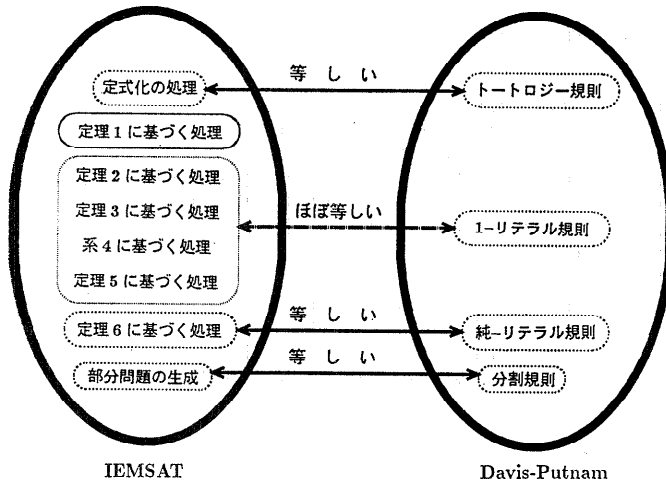
図2 IEMSAT と Davis-Putnam の関係
