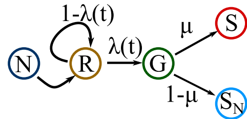
図2 状態遷移図
