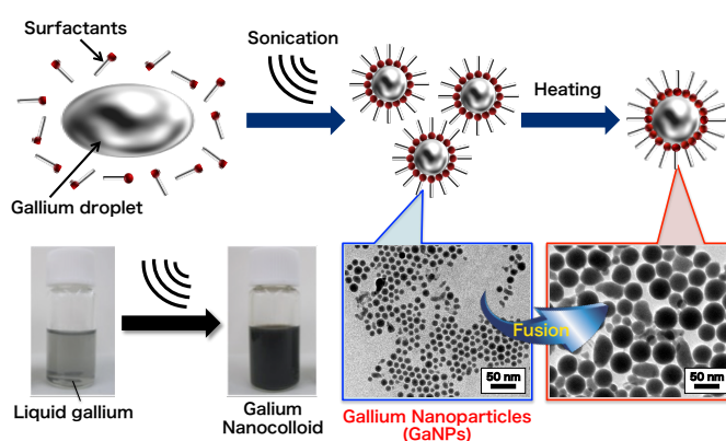
図 1. GaNPs の作製及び融合挙動の概念図と TEM 像。
