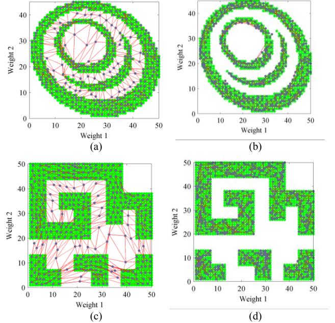
Fig. 3. Experimental results. (a) SOM on data set 1. (b) SOM on data set 2. (c) REISOD on data set 1. (d) REISOD on data set 2.
