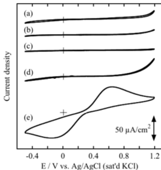
図2 (a) CH 3 -TM、(b) OH-TM、(c) NH 2 -TM、(d) COOH-TM をそれぞれ修飾した HOPG 電極と (e) 未修飾 HOPG 電極の 1 mM K 4 [Fe(CN) 6 ] を含む 0.1 M KCl 水溶液の酸化還元応答 (掃引速度 100 mV·s -1 )。
