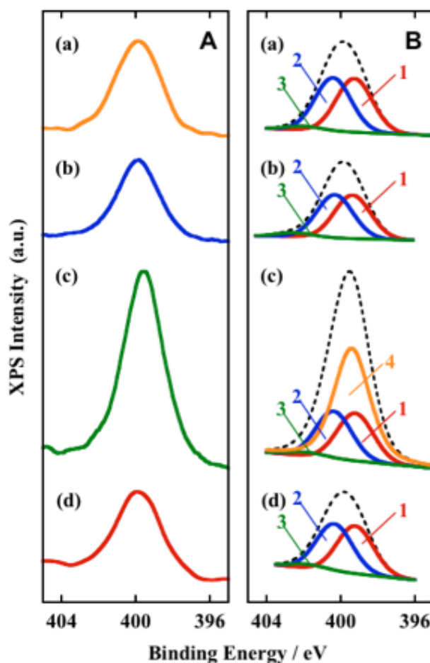
図 1 (A) (a) \text{CH}_3\text{-TM} 、(b) \text{OH-TM} 、(c) \text{NH}_2\text{-TM} 、(d) \text{COOH-TM} をそれぞれ修飾した HOPG 電極の XPS N1s スペクトル。(B) XPS N1s スペクトルをピーク分離した結果と分離スペクトルの和（点線）で、1 は \text{C-NH-C} （第二級アミン）、2 は水素結合した \text{C-NH-C} 、3 はプロトネーションした \text{C-NH}_2^+\text{-C} 、4 は \text{C-NH}_2 （第一級アミン）由来のスペクトルである。
