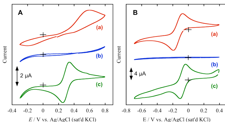
図 6 (a) CH 3 -TM 構築前と(b)構築後のグラフェン/Au(111)単結晶電極、(c) 0.1 M LiClO 4 水溶液で電解酸化を行ったグラフェン/Au(111)単結晶電極のサイクリックボルタモグラム。それぞれの測定条件は(A) 2 mM K 4 [Fe(CN) 6 ]を含む 0.1 M KCl 水溶液、掃引速度:10 mV·s -1 、(B) 1 mM [Ru(NH 3 ) 6 ]Cl 3 を含む 0.1 M KCl 水溶液、掃引速度:100 mV·s -1 。
