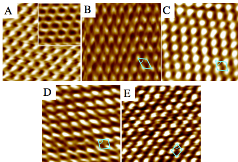
図 3 A:未修飾 HOPG 電極および、B:CH 3 -TM、C : OH-TM、D : NH 2 -TM、E : COOH-TM をそれぞれ修飾した HOPG 電極の STM 像および単位格子(STM 像のサイズは 2 nm × 2 nm)。
