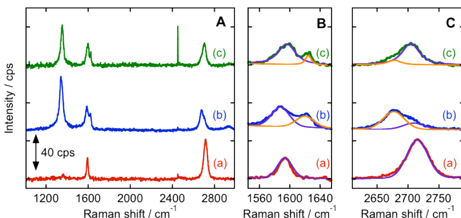
図5(A) (a) グラフェン/Au(111)単結晶電極と(b) \text{CH}_3 -TM 構築グラフェン/Au(111)単結晶電極、(c) 0.1 \text{ M LiClO}_4 水溶液で電解酸化したグラフェン/Au(111)単結晶電極のラマンスペクトル。(B)および(C)はそれぞれのスペクトルの G band 領域、2D band 領域をピークフィッティングしたもので、紫色は構築前から観測されるバンドを、橙色は \text{CH}_3 -TM 構築後に新たに観測されたバンドである。
