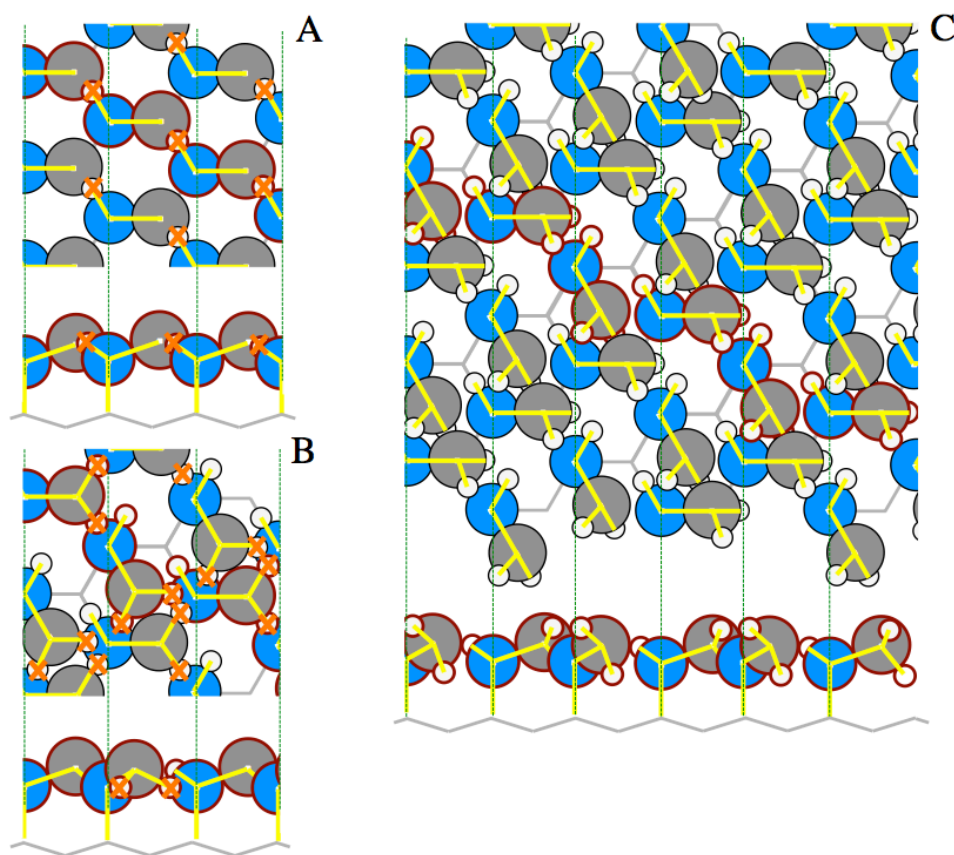
図 4 基板のグラファイト構造と表面上に構築されたアルキルアミンの上面方向(上)と側面方向(下)から見た修飾モデル。(A)アルキルアミンが同一配向で修飾された修飾モデル、(B)原子の重なりを解消するためにグラファイトの炭素原子と窒素原子間の C-N 結合を軸に 60°回転させた修飾モデル、(C) \alpha 炭素原子に付属した水素原子と窒素原子の重なりを解消させるために \alpha 炭素原子と窒素原子間の C-N 結合を軸に 60°回転させた修飾モデル。
