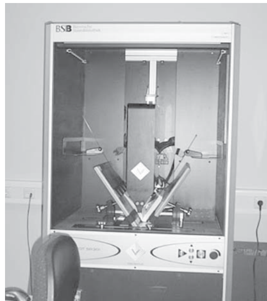
バイエルン州立図書館のデジタル化センターで使用されているブックスキャナ「ScanRobot」
