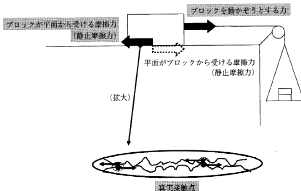
図5 静止摩擦力・物体を動かそうと加える力・真実接点の関係
