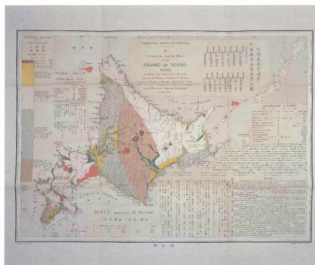
ラインマンが編集した北海道の地質図 広域な総合地質図としては、日本最初の地図である と言われている。
