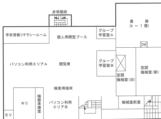
4 階
