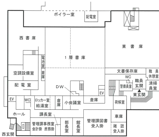
1 階
