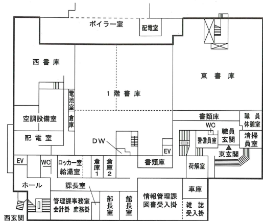
1 階
