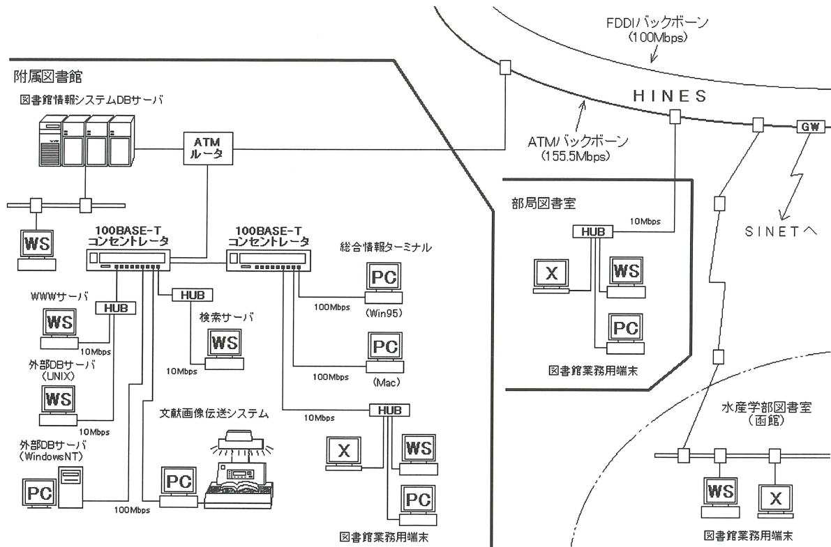
北海道大学附属図書館ネットワーク構成図（平成 9 年 4 月）
