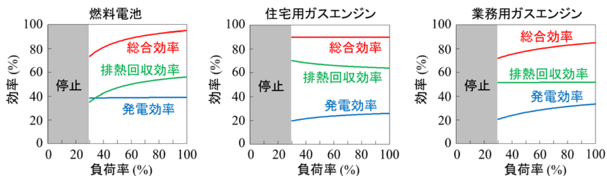
各種コジェネ機種の効率曲線
