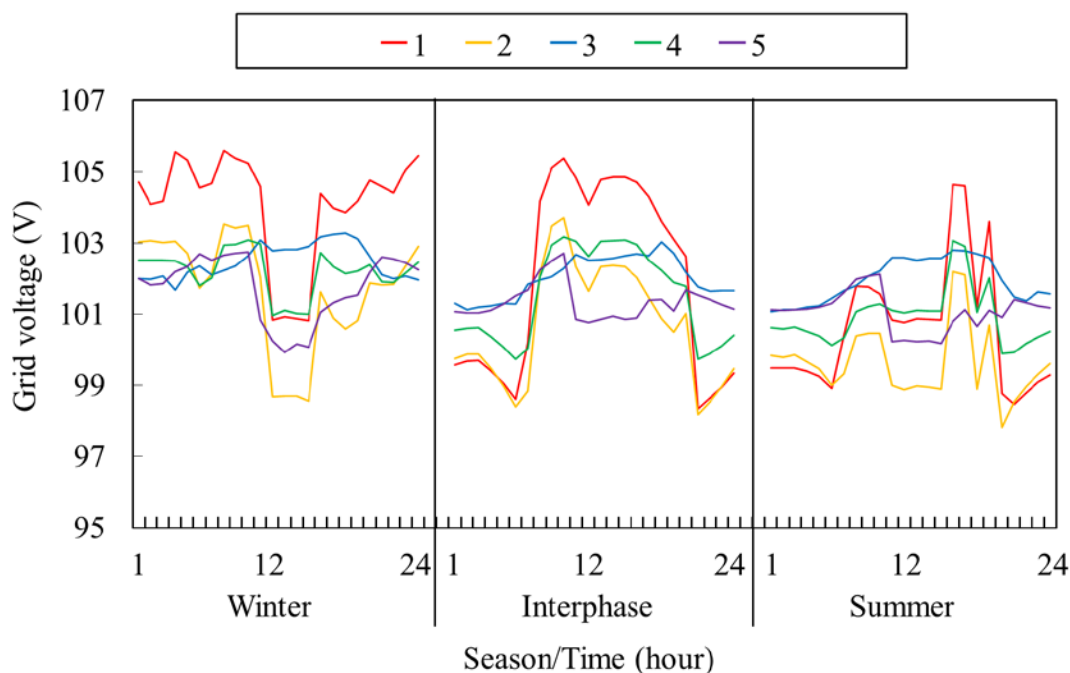
図 3.8 各配電線における需要端電圧
