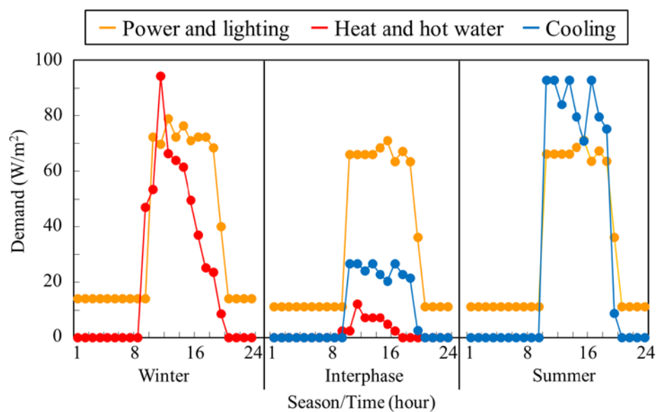
図 2.4(d) 北海道の店舗における単位床面積あたりの需要パターン
