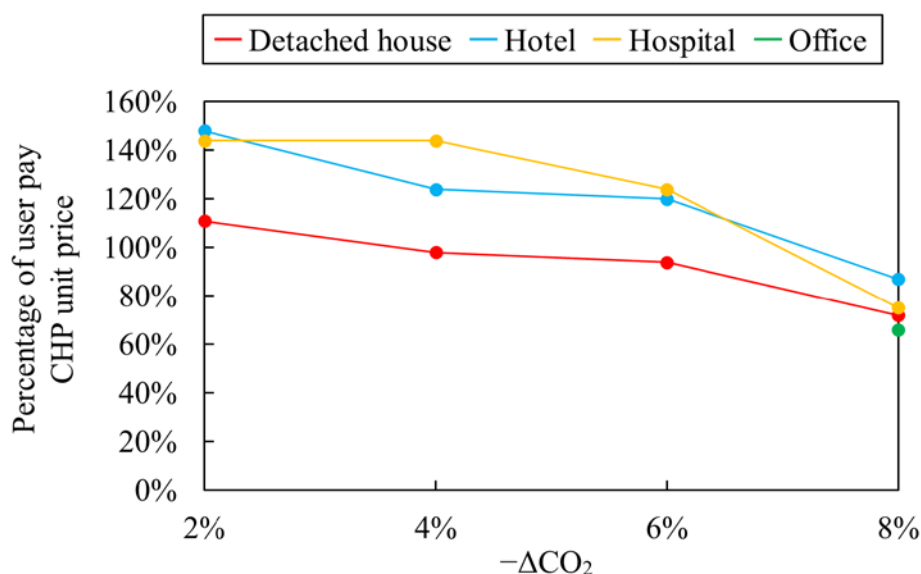
図 5.6 各 \text{CO}_2 削減率において需要家選択を社会最適な設備量構成に誘導するためのコジェネ設備価格条件
