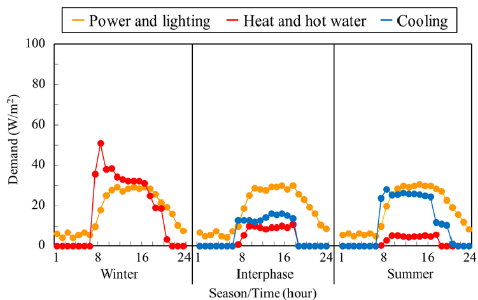
図 2.4(e) 北海道の事務所における単位床面積あたりの需要パターン
