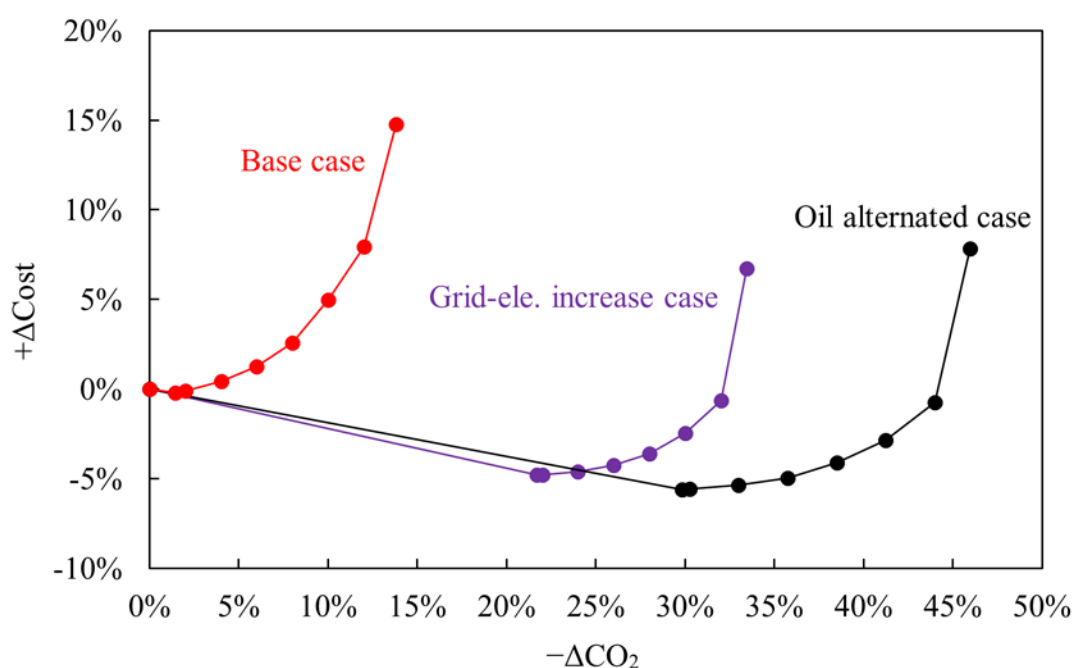
図 3.10 コジェネの電力を石油火力代替と想定した場合の影響
