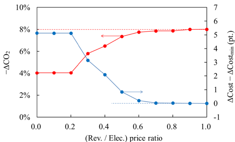
図 5.3 逆潮流買取／電力価格比が CO 2 削減率ならびに追加社会コストに与える影響（設備量構成：CO 2 削減率 8%）
