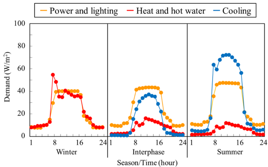
図 4.6(c) 東京の病院における単位床面積あたりの需要パターン
