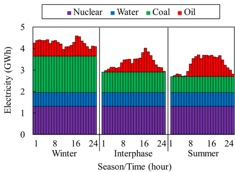
図 B.1 系統電力の電源構成
