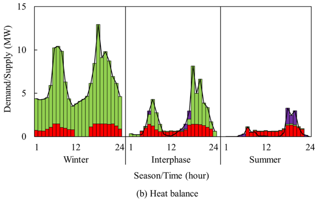
図 3.4 コスト増加率 5%時の独立型の戸建住宅における (a) 電力と (b) 熱のエネルギーバランス
