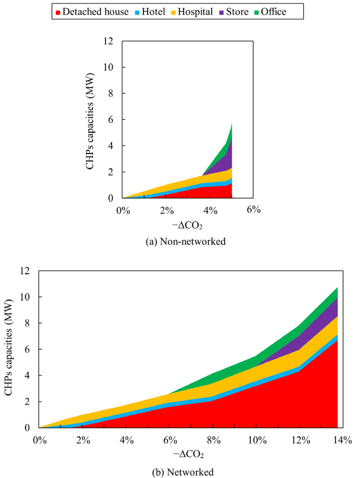
図 3.3 (a) 独立型ならびに (b) 分散協調型におけるコジェネの設備量
