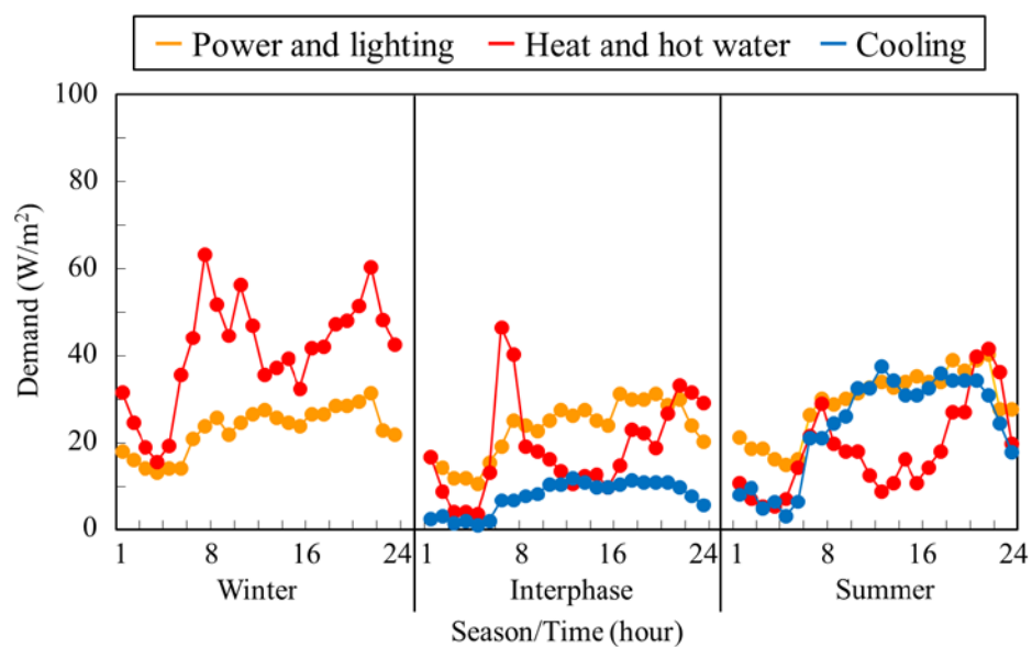
図 2.4(b) 北海道のホテルにおける単位床面積あたりの需要パターン
