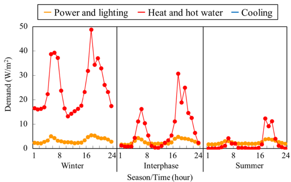
図 2.4(a) 北海道の住宅における単位床面積あたりの需要パターン
