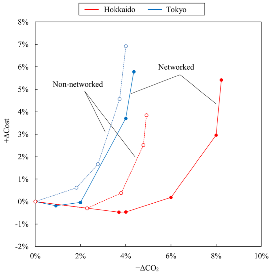
図 4.10 北海道と東京の都市住宅地区において戸建住宅にガスエンジンを導入した場合の独立型と分散協調型の \text{CO}_2 -コスト曲線
