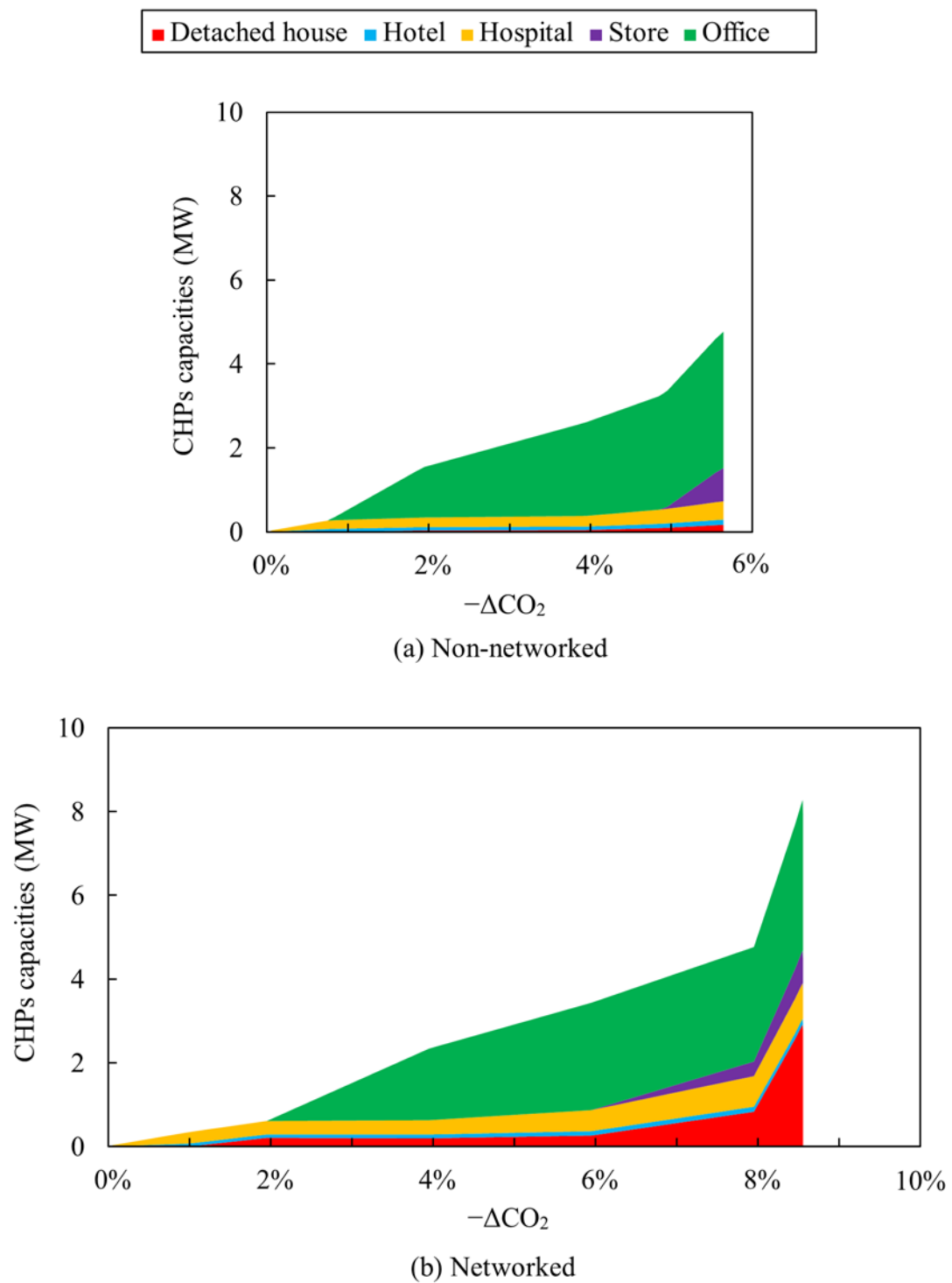
図 4.4 都市商業地区の (a) 独立型ならびに (b) 分散協調型におけるコジェネ設備量
