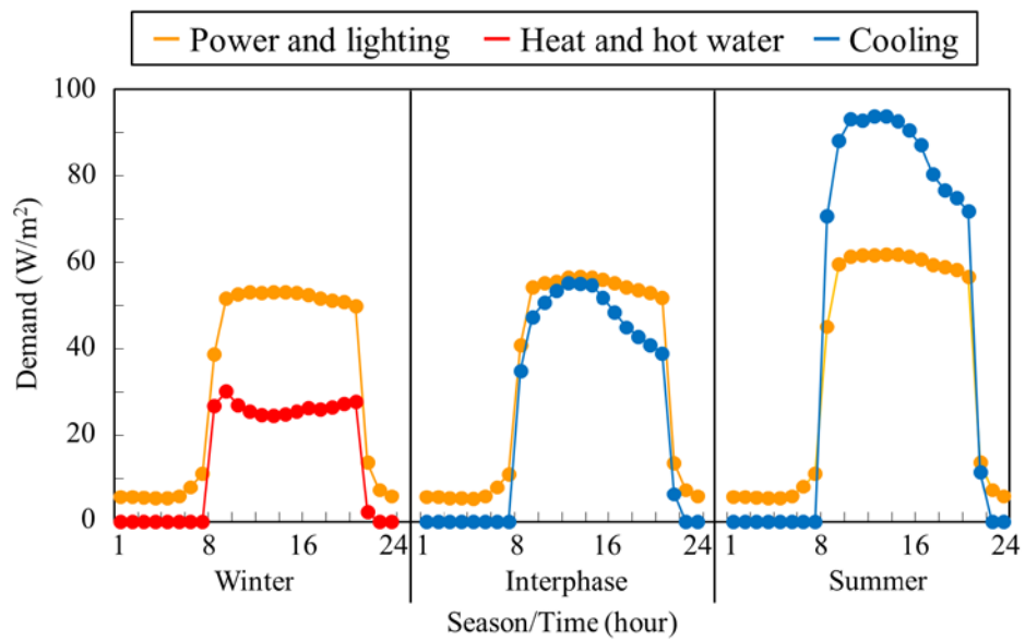
図 4.6(d) 東京の店舗における単位床面積あたりの需要パターン
