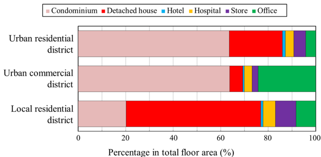
図 2.3 各地区における各種建物の延床面積割合
