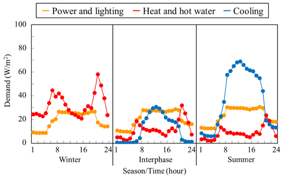
図 4.6(b) 東京のホテルにおける単位床面積あたりの需要パターン
