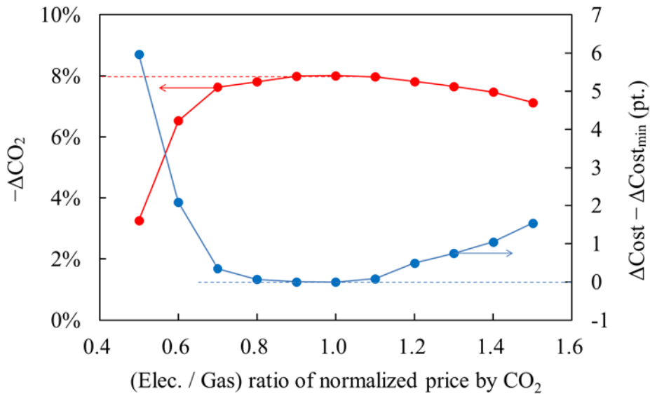
図 5.2 電力／ガス価格比が CO 2 削減率ならびに追加社会コストに与える影響（設備量構成：CO 2 削減率 8%）
