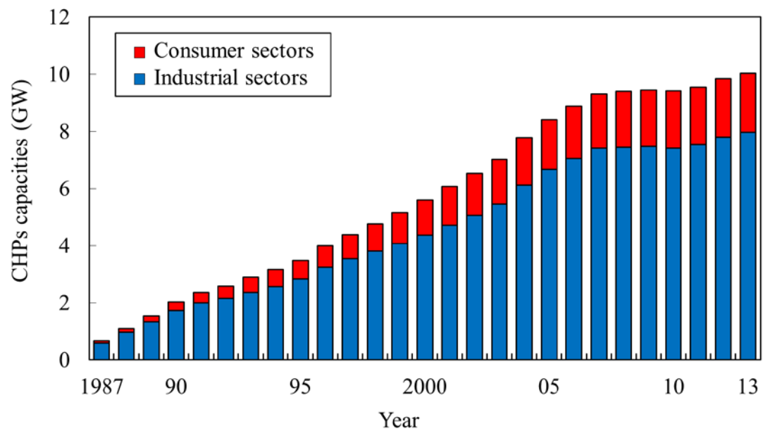
図 1.3 日本におけるコジェネレーションの設備容量の推移 出典：エネルギー白書 2015 (経済産業省, 2015) を基に作成 原典：コジェネ導入実績報告 (コージェネ財団, 2014)
