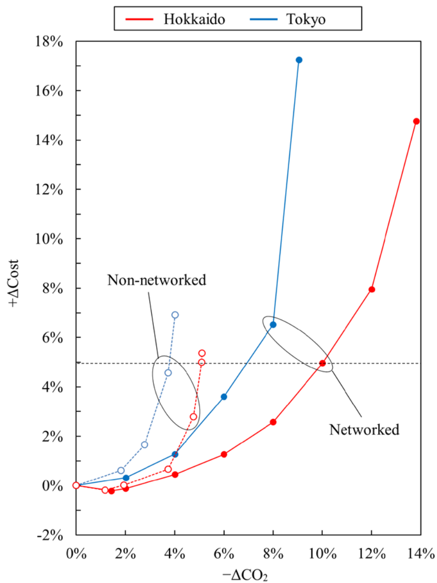
図 4.9 北海道と東京の都市住宅地区において戸建住宅に燃料電池を導入した場合の独立型と分散協調型の \text{CO}_2 -コスト曲線
