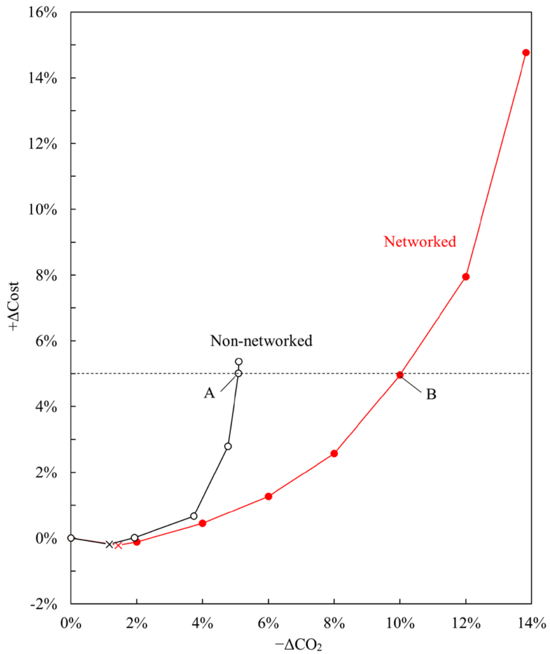
図 3.2 独立型と分散協調型の \text{CO}_2 -コスト曲線
