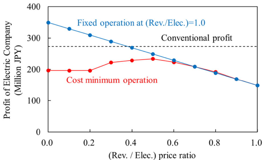
図 5.4 電力会社の利益に対する逆潮流買取／電力価格比影響
