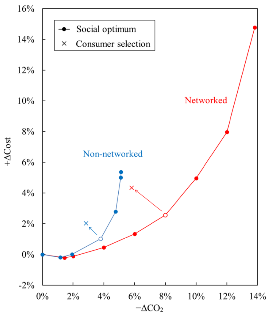
図 5.1 CO 2 －コスト曲線（社会最適）ならびに需要家選択
