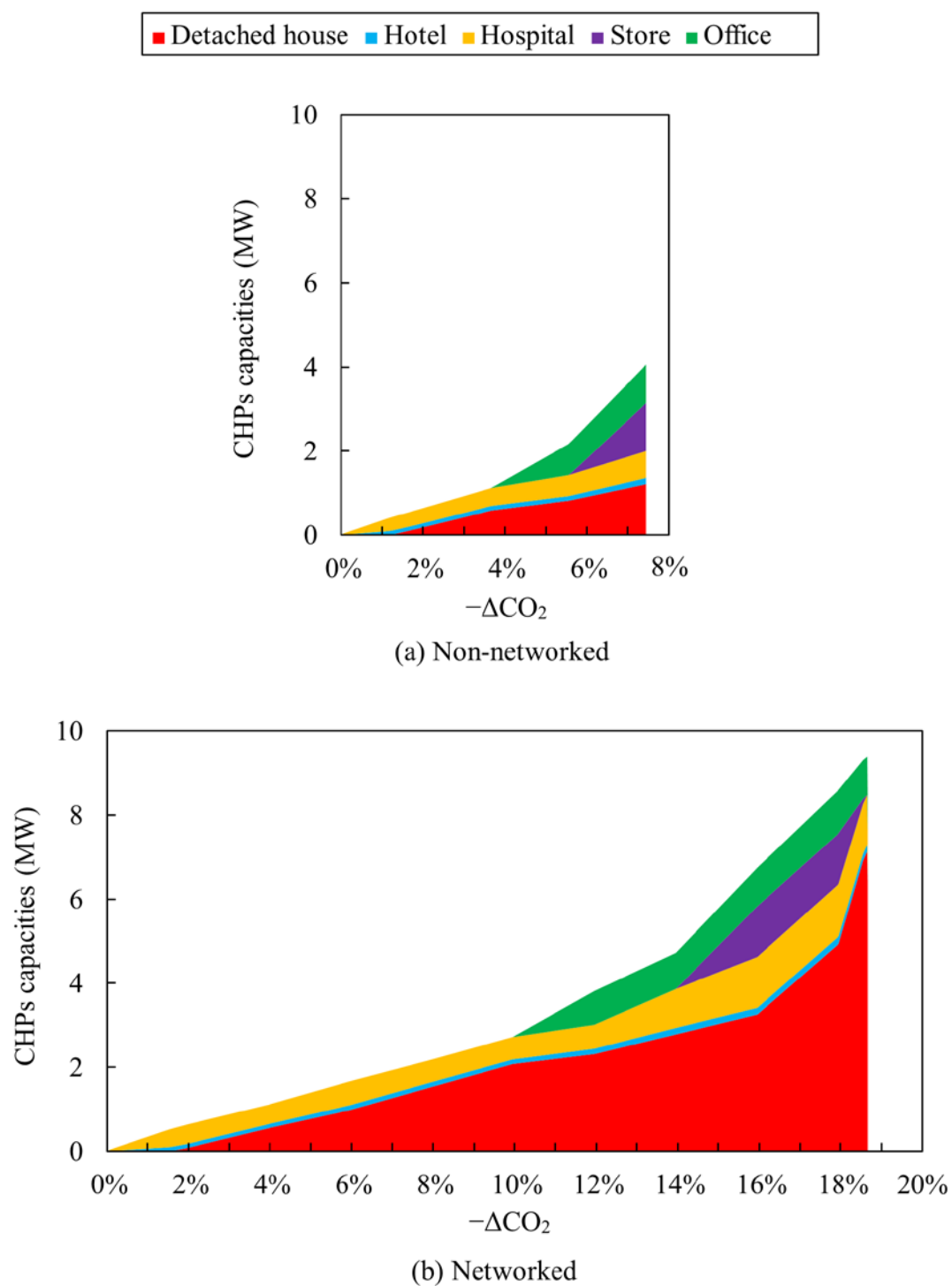
図 4.5 地方住宅地区の (a) 独立型ならびに (b) 分散協調型におけるコジェネ設備量
