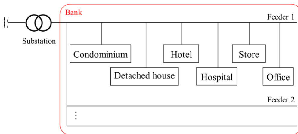
図 2.1 解析対象地域のモデル化
