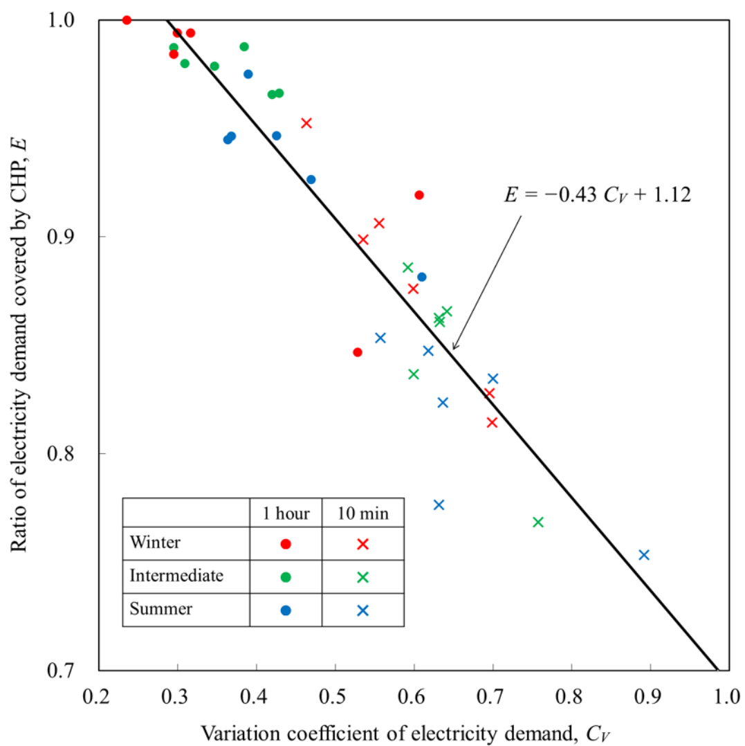
図 3.1 電力需要の変動係数に対する，全電力需要に占める コジェネの発電量の割合
