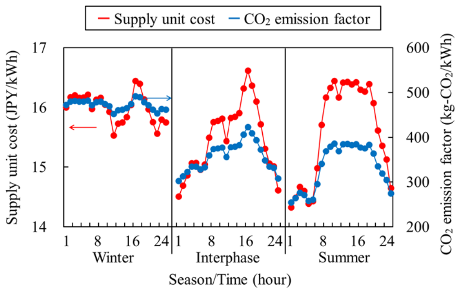
図 B.2 系統電力の供給原価ならびに CO 2 排出原単位
