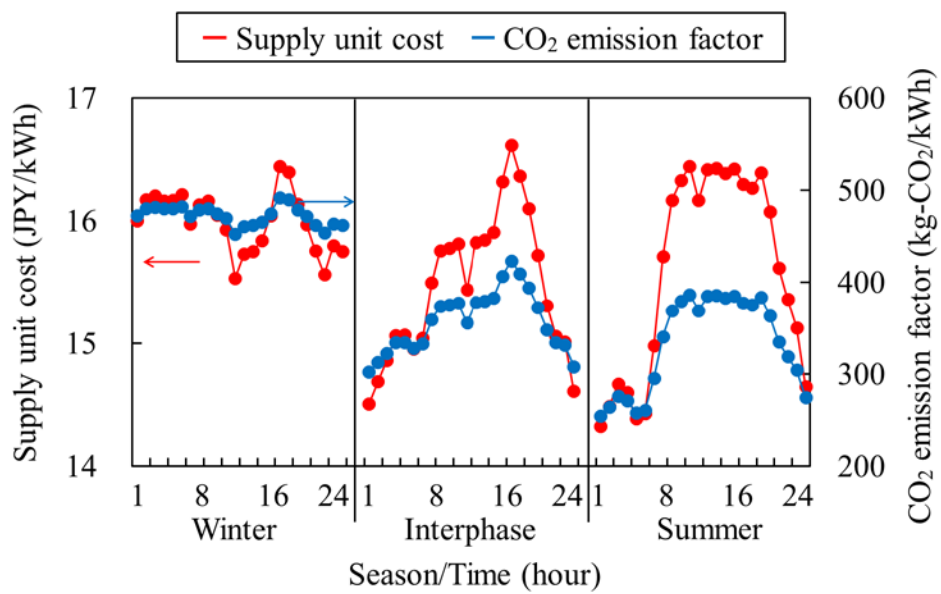
図 2.7 系統電力の供給原価ならびに CO 2 排出原単位
