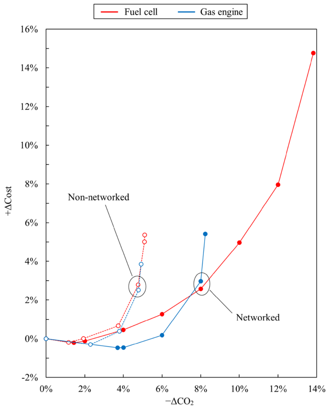
図 4.7 ベースケースにおいて戸建住宅のコジェネを燃料電池または住宅用ガスエンジンとしたときの独立型と分散協調型の CO 2 －コスト曲線
