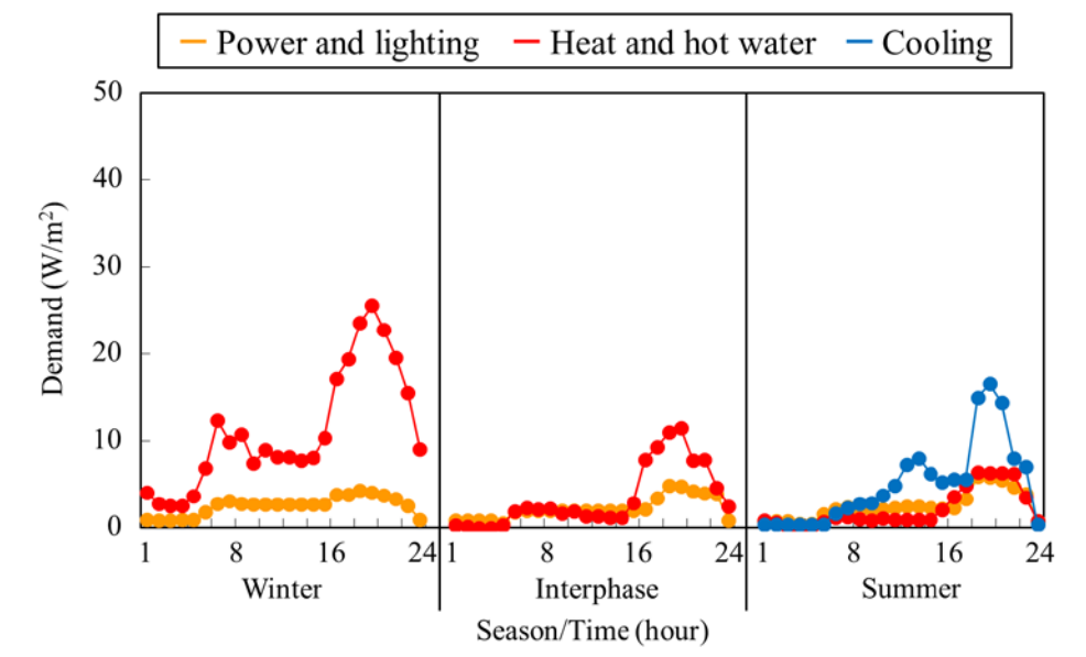
図 4.6(a) 東京の住宅における単位床面積あたりの需要パターン
