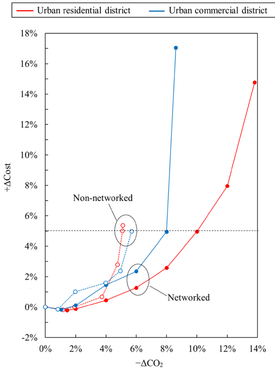
図 4.1 都市商業地区および都市商業地区における 独立型と分散協調型の CO 2 -コスト曲線
