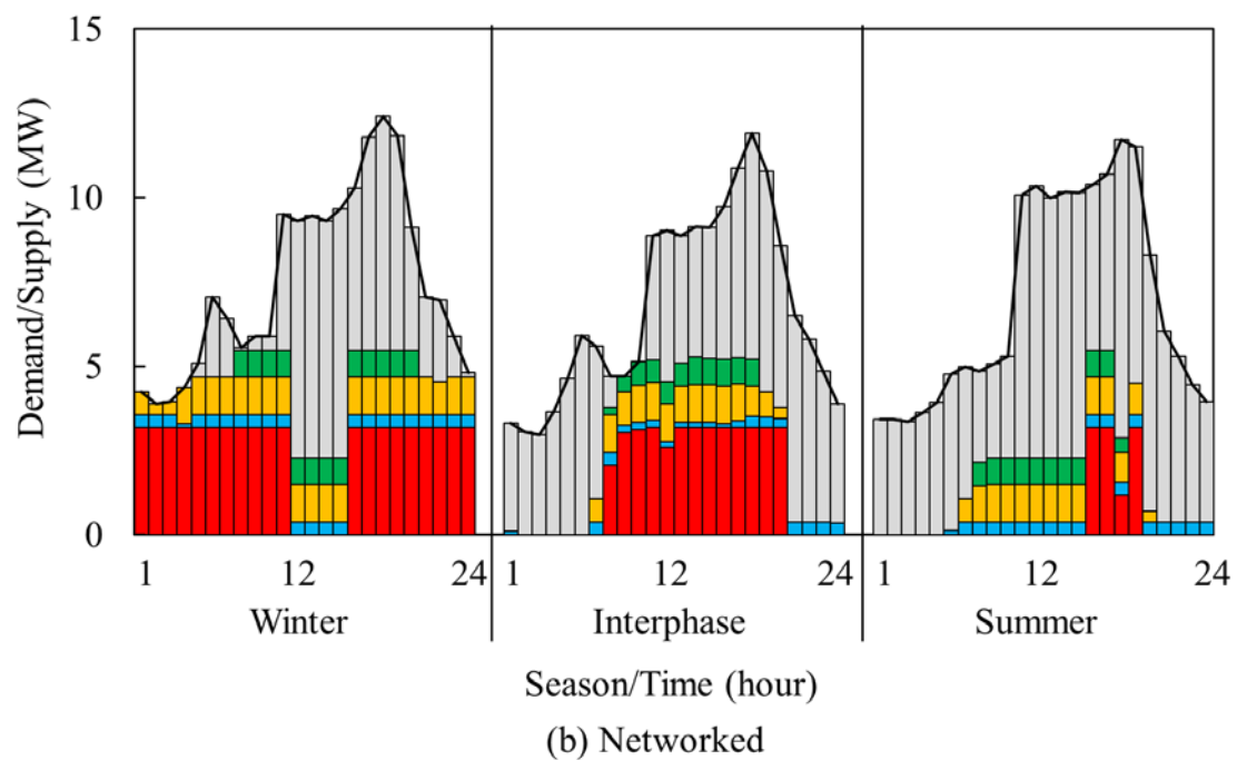
図 3.7 コスト増加率 5%時の (a) 独立型と (b) 分散協調型における対象地域全体の電力のエネルギーバランス
