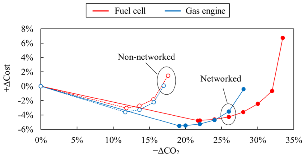
図 4.8 系統増加ケースにおいて戸建住宅のコジェネを燃料電池または住宅用ガスエンジンとしたときの独立型と分散協調型の \text{CO}_2 －コスト曲線
