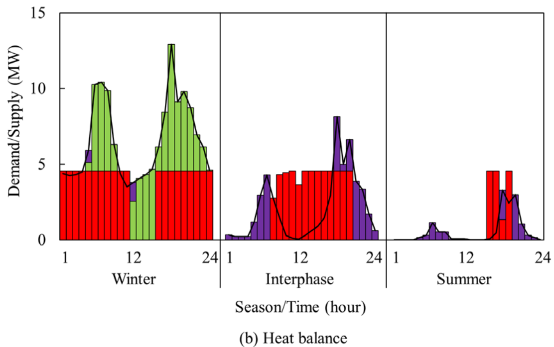
図 3.6 コスト増加率 5%時の分散協調型の戸建住宅における (a)電力と(b)熱のエネルギーバランス
