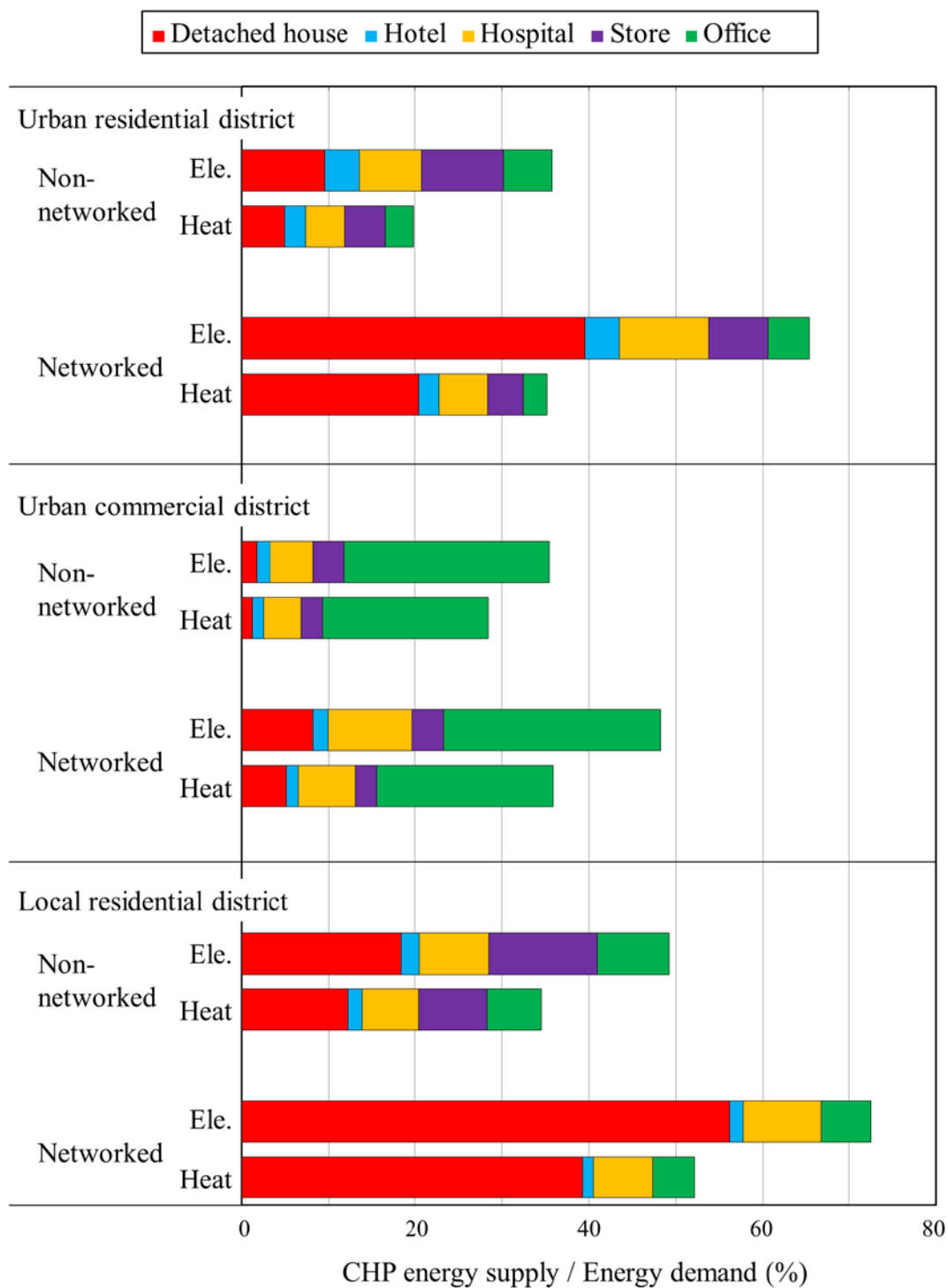
図 4.3 最高 CO 2 削減率時の各地域における電力ならびに熱需要に対するコジェネのエネルギー供給割合
