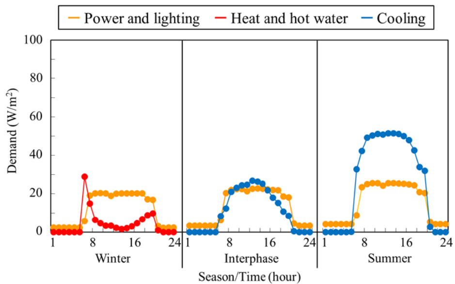
図 4.6(e) 東京の事務所における単位床面積あたりの需要パターン
