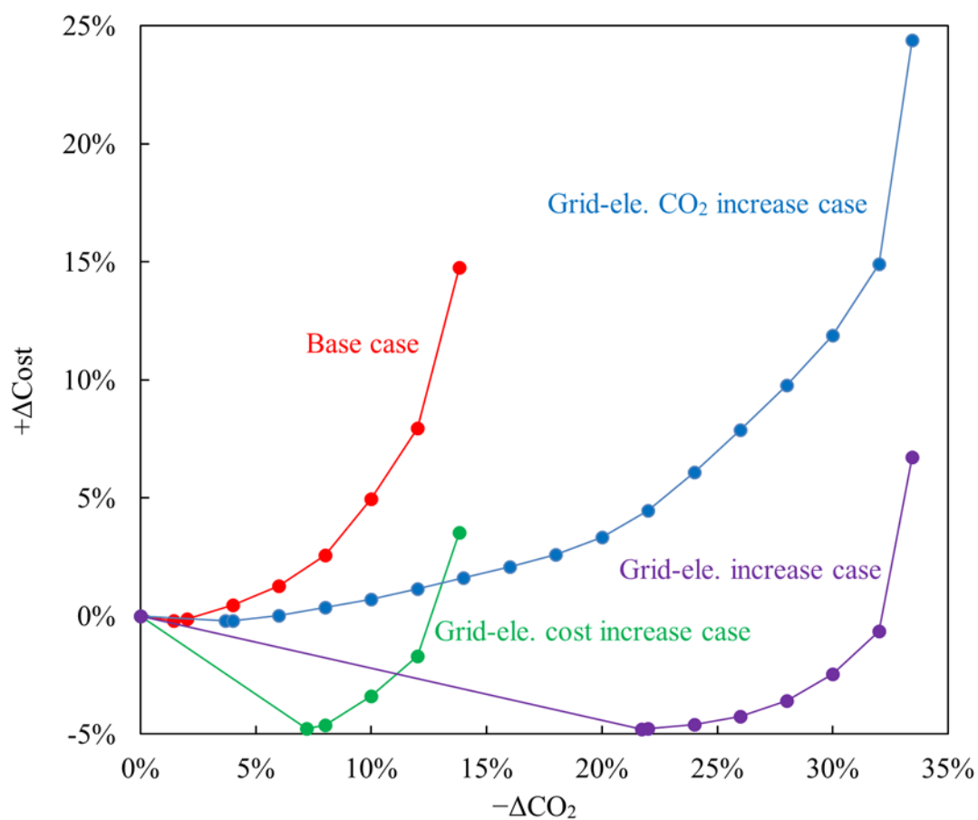
図 3.9 CO 2 -コスト曲線の感度分析
