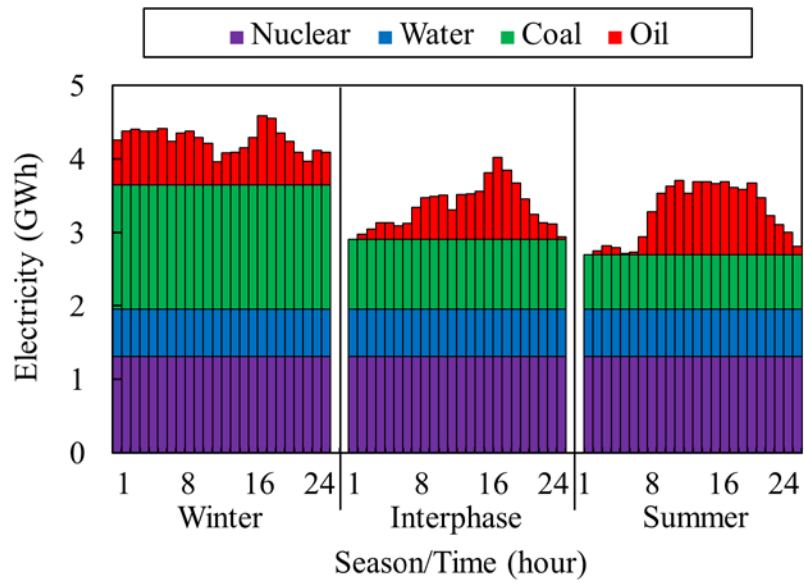
図 2.6 系統電力の電源構成
