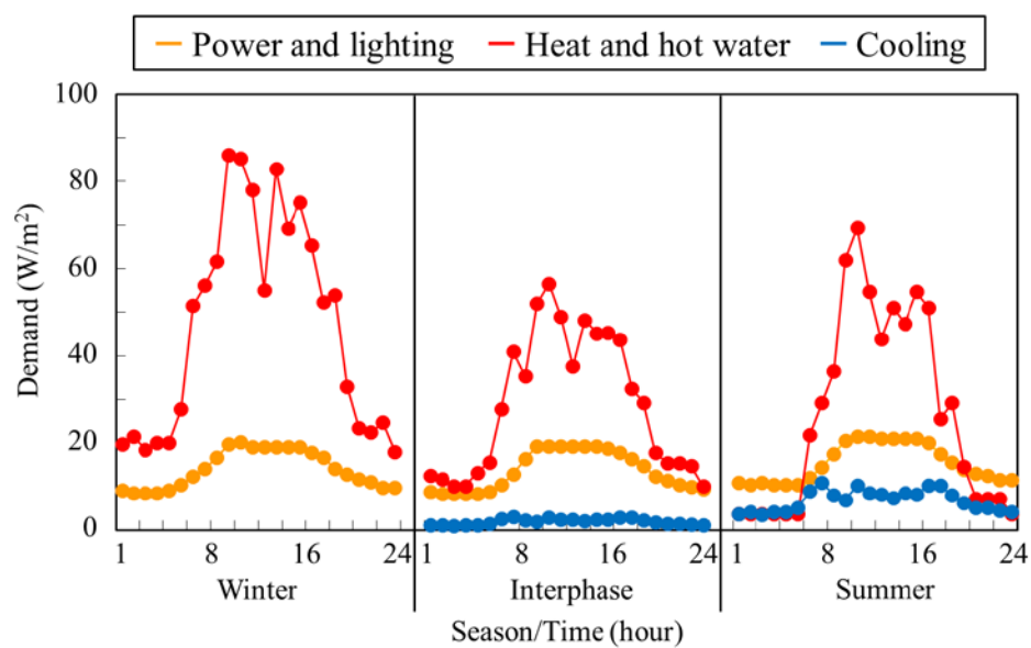
図 2.4(c) 北海道の病院における単位床面積あたりの需要パターン
