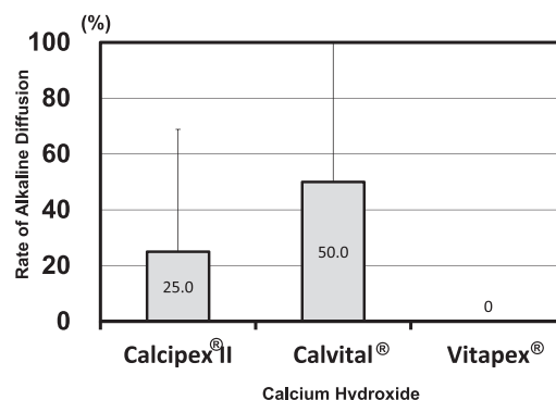
Fig. 10 Rate of ion diffusion
