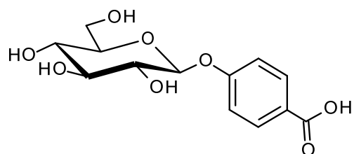
p -SAG
