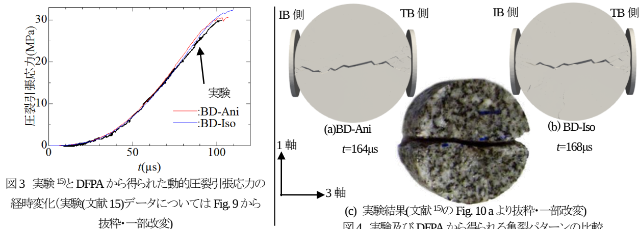
図 4 実験及び DFPA から得られる亀裂パターンの比較
