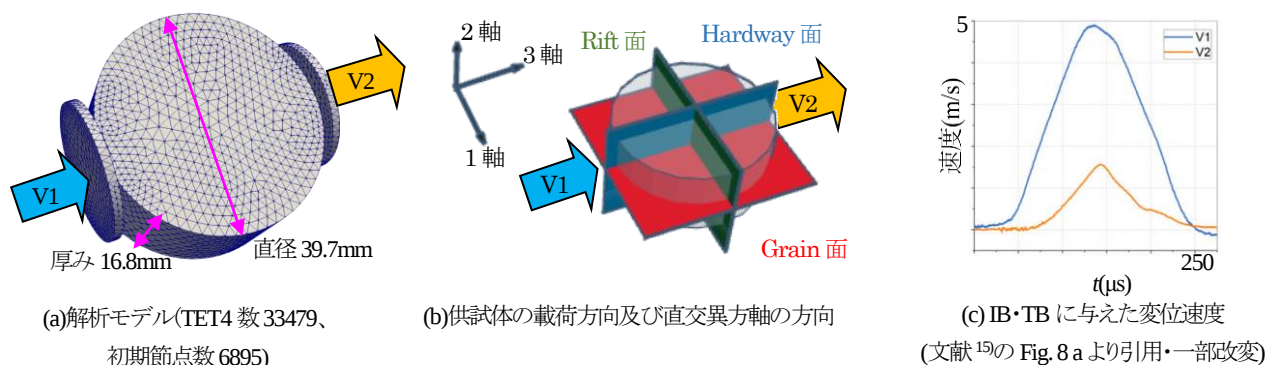
図 2 Bare 花崗岩の動的圧裂引張試験を模擬した解析の概要
