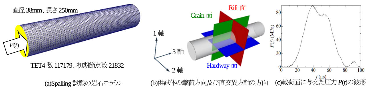
図 6 Spalling 試験の解析モデルの概要
