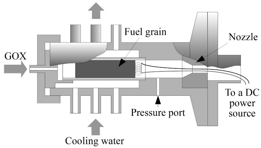
Fig. 4 Test motor.
