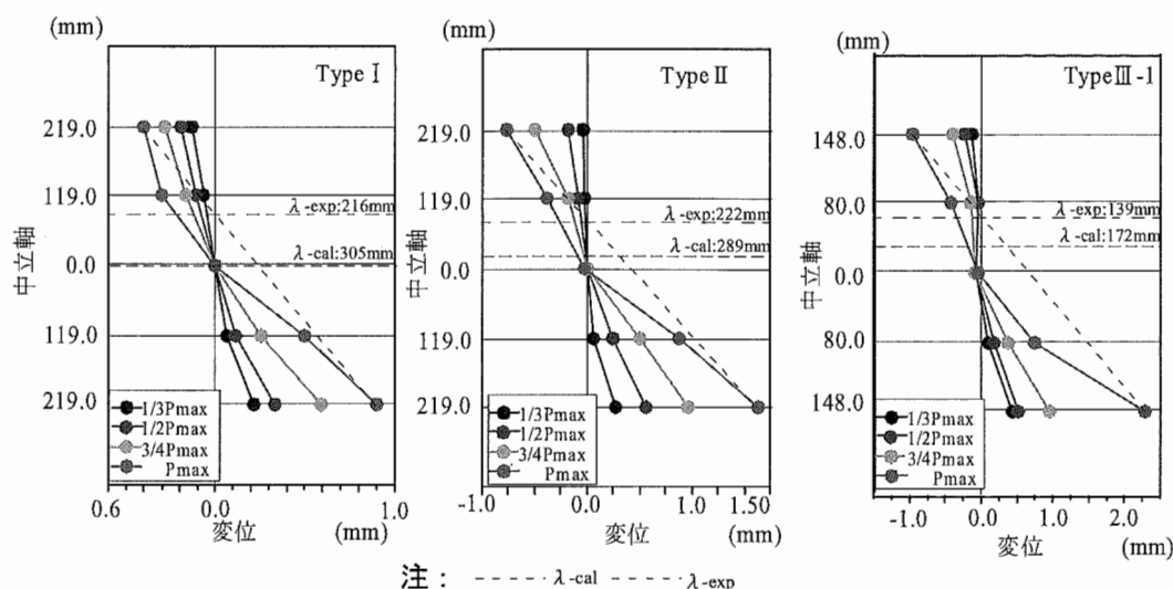
第7図 中立軸と各荷重域での変位量
