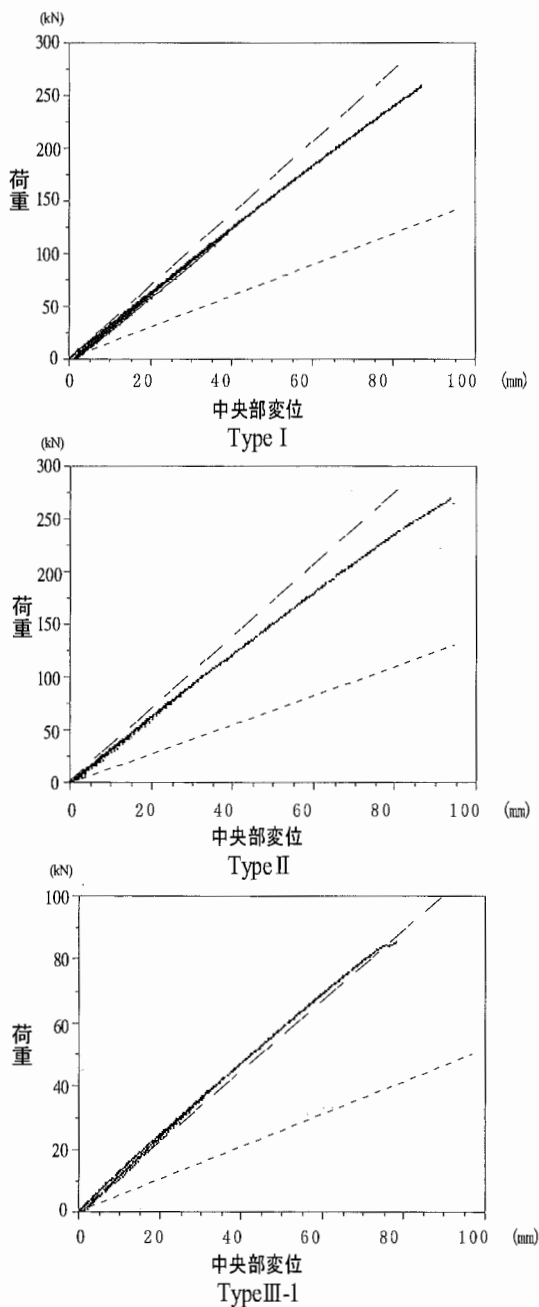
注 ----- : (18) 式による計算値 \delta_m - - - - - : (18) 式による計算値 \delta_b 第6図 各たわみ計算値との関係
