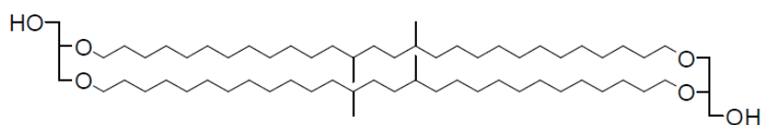
GDGT I (1022)
