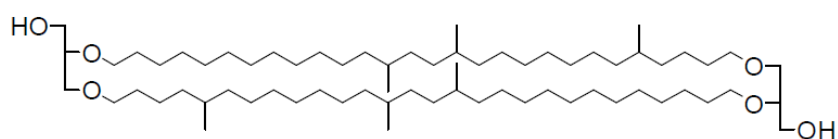
GDGT III (1050)
