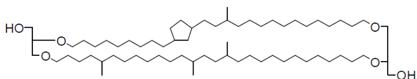
GDGT IIb (1034)
