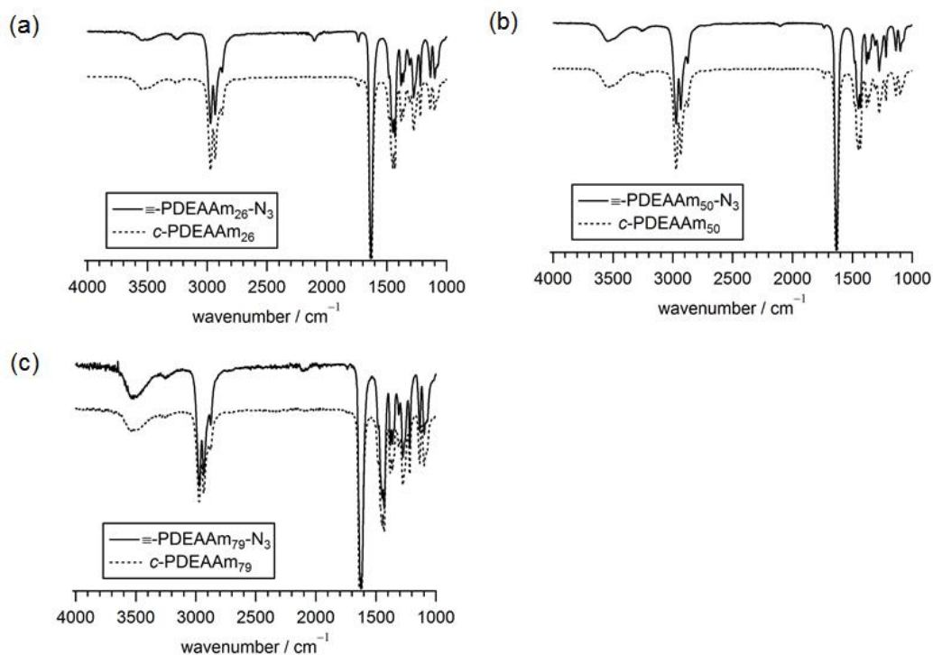
Figure 3-9. FT-IR spectra of \equiv -PDEAAm- N_3 and c -PDEAAm.
