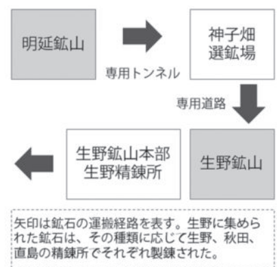
■図2 鉱山稼働時の産出から精錬までの流れ（出所）筆者作成
