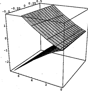
cuspidal edge
