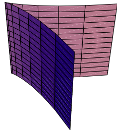
cuspidal edge
