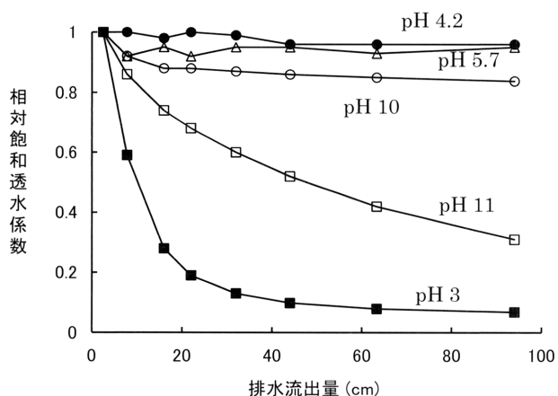
図4 アロフェン質火山灰土の飽和透水係数に及ぼす 1 \text{ mol} \cdot \text{L}^{-1} 塩化ナトリウム (Na-H-Cl-OH 系) 浸透溶液 pH の影響 (Ishiguro, 2005 を一部改図)
