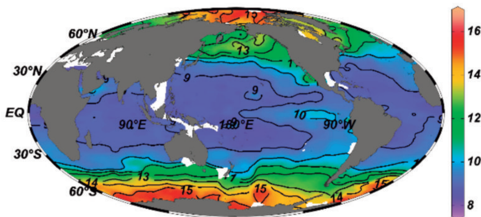
図2：表層海水のルベール係数。GLODAP-v2.1 データセット (Olsen et al., 2016) に含まれる 1973-1999 年の観測データを用いて算出。
