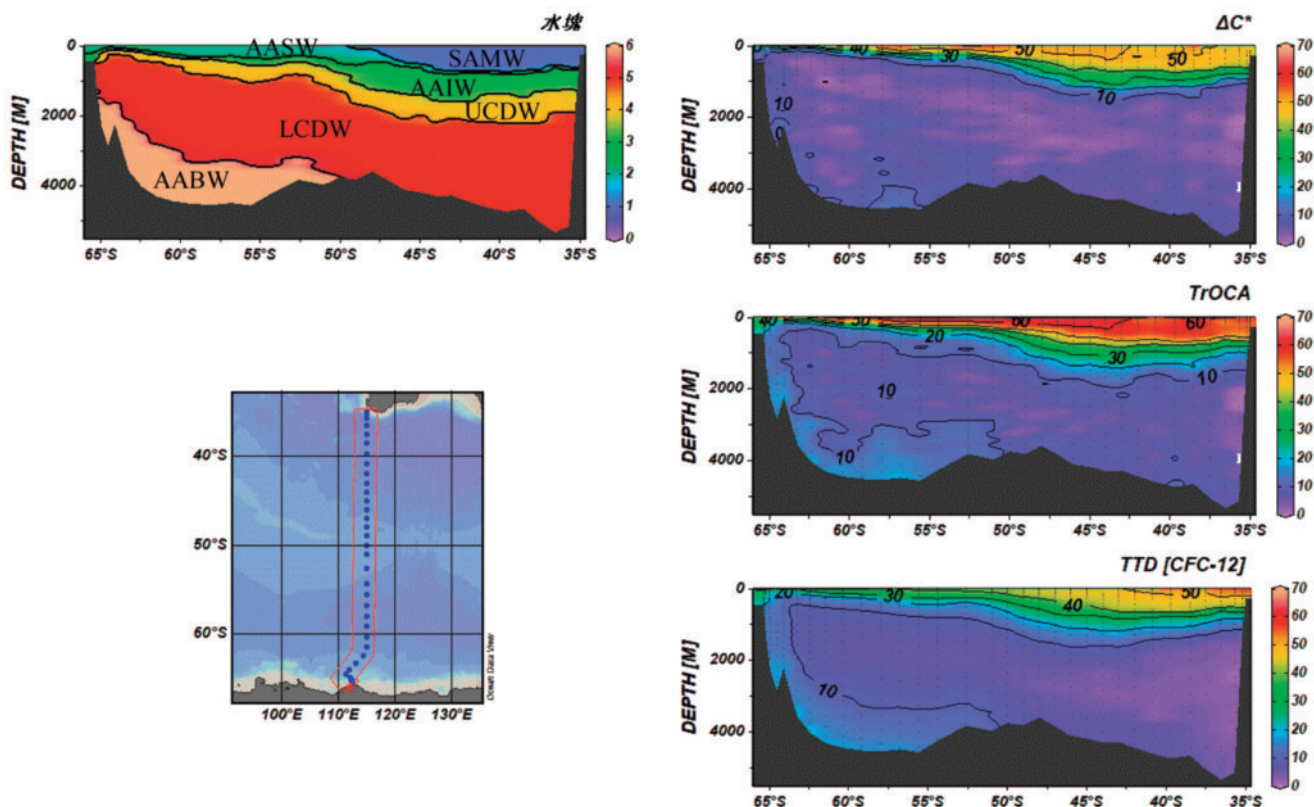
図7：南大洋オーストラリア南部（左下の観測ライン沿い）における観測ベースの人為起源CO 2 の見積もり例（橋本，2018；観測データはGLODAP-v2.1データセットから）。右は上からΔC*法，TrOCA法，TTD法（CFC-12）の結果。単位はμmol kg -1 。左上はCarter et al. (2008)を参考に分類した水塊分布を示す（濃青：亜南極モード水（SAMW），薄青：南極表層水（AASW），緑：南極中層水（AAIW），黄：周極深層水上部（UCDW），赤：周極深層水下部（LCDW），桃：南極底層水（AABW））。
