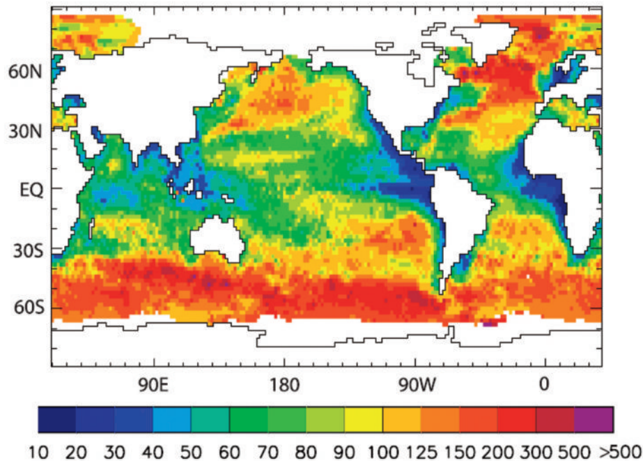
図4：各海域における年間最大混合層深度（m）。de Boyer Montégut et al. (2004) から改変。
