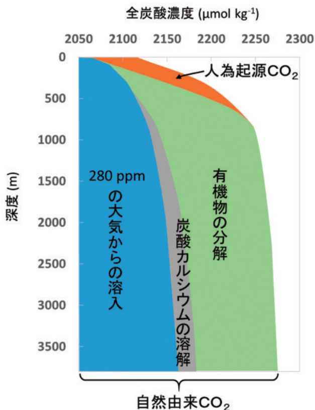
図5：全炭酸の鉛直分布とその濃度を支配する要因（野崎, 1994 を参考に作図）。南大洋（50° S, 115° E）の例を示す。青色は 280 ppm の大気との平衡にあった時の全炭酸濃度で、水温・塩分・アルカリ度によって変化する。灰色、緑色、橙色はそれぞれ、炭酸カルシウムの溶解、有機物の分解、人為起源 \text{CO}_2 によって増加した全炭酸。2005 年の観測データから算出。
