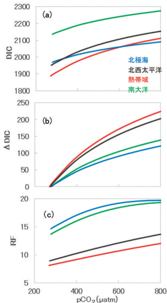
図3：大気中 \text{CO}_2 分圧を産業革命以前の値から上昇させたときの (a) 海水中全炭酸濃度の変化、(b) 産業革命以前からの全炭酸濃度の増加量、(c) RF の変化。青：北極海 (31, 0°C, 2100 \mu\text{mol kg}^{-1} )、黒：北西太平洋 (34, 22°C, 2300 \mu\text{mol kg}^{-1} )、赤：熱帯域 (35, 28°C, 2300 \mu\text{mol kg}^{-1} )、緑：南大洋 (34, 0°C, 2300 \mu\text{mol kg}^{-1} )。カッコ内に示した海域ごとの代表的な塩分、水温、アルカリ度を用い、常に大気と平衡状態にあると仮定して計算。
