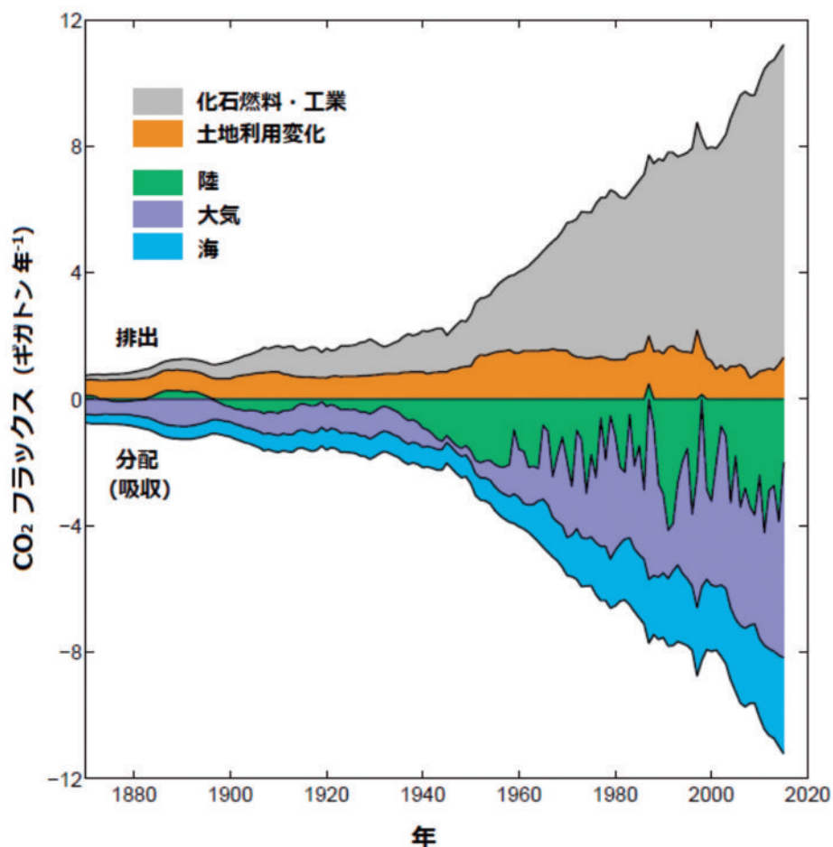
図1：1870年から2016年までのCO 2 排出量と吸収量の経年変化。Le Quéré et al. (2016) を改変。
