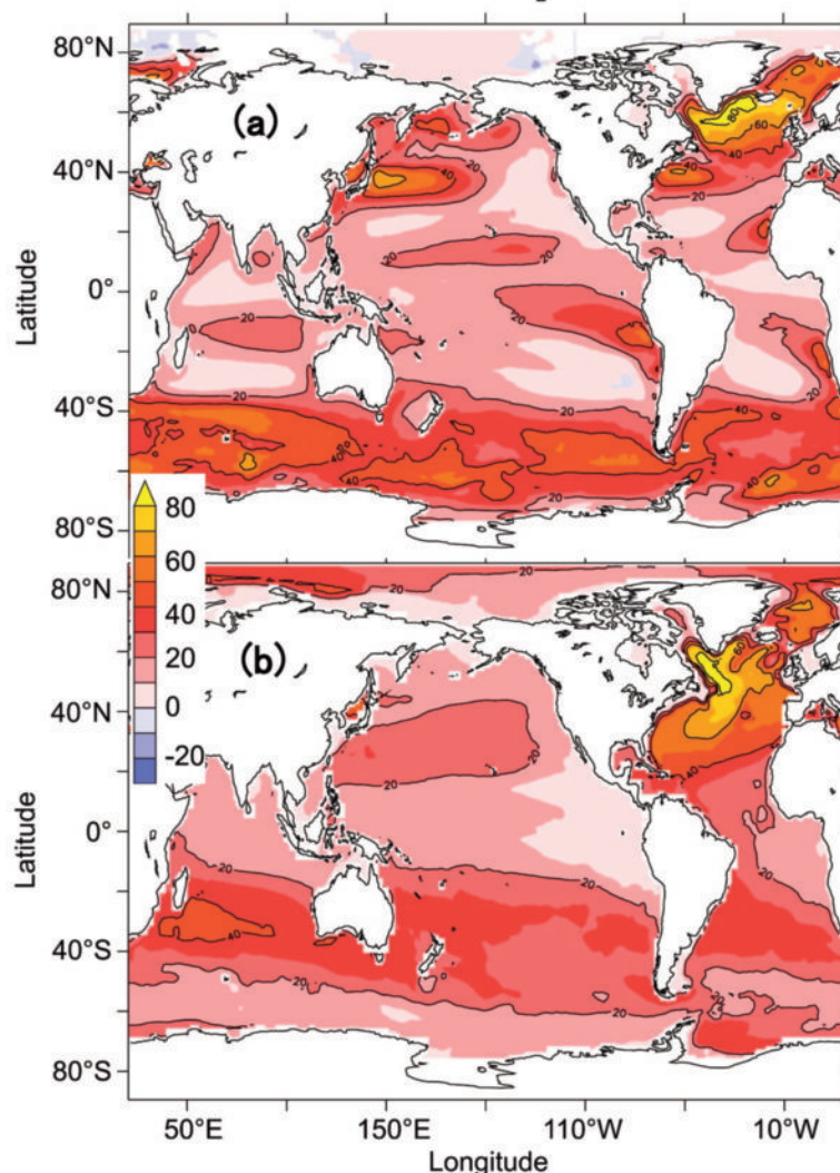
図6：人為起源CO 2 の(a)表層での取り込み量と(b)存在量(1970年から1995年までの積算値)。モデルシミュレーションの結果。単位はmol m -2 。Frölicher et al. (2015)の図を改変。
