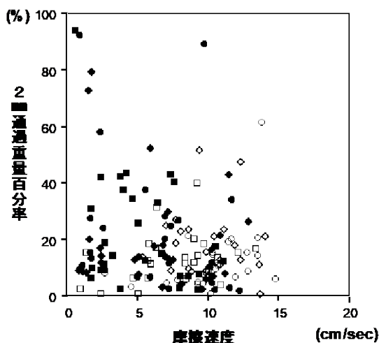
図－１ 底質中の2 mm通過重量百分率と摩擦速度との関係。黒塗は瀬，白塗は平水時を示す。（山田 2002に加筆修正）。
