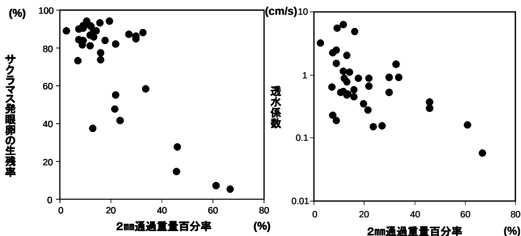
図ー4 サクラマス発眼卵の生残率と底質中の2 mm通過重量百分率および透水係数との関係(山田 2002 に加筆修正).
