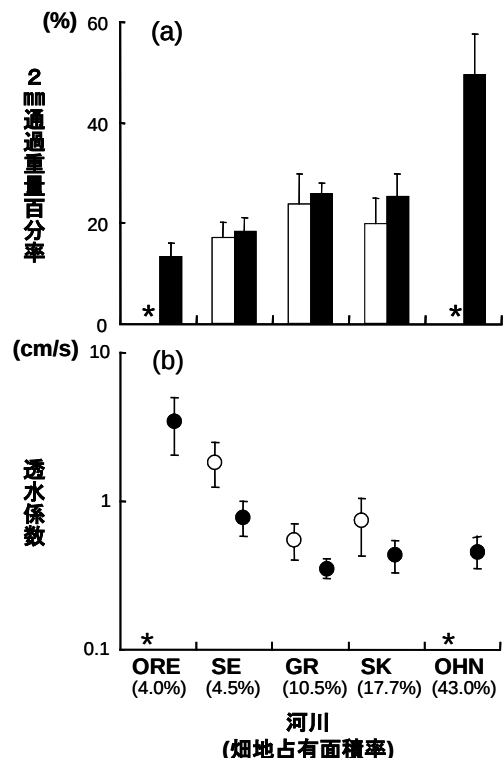
図－２ 流域の畑地占有面積率の異なる河川における(a)底質中の2 mm通過重量百分率および(b)透水係数の平均値と標準誤差。黒塗は出水直後，白塗は平水時を示す。*は欠測値を示す(村上ら 2001に加筆修正)。
