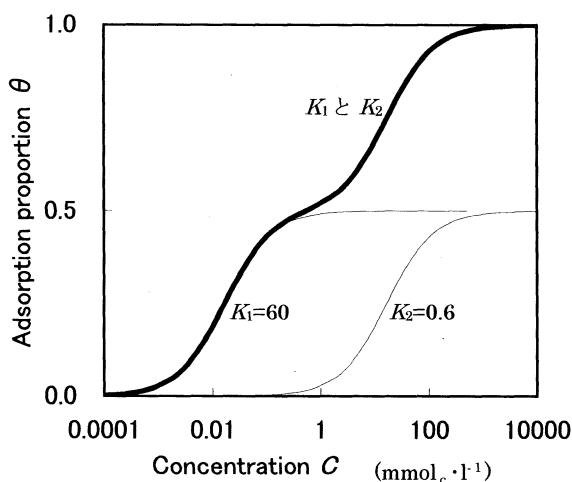
Fig.1 ラングミュアの式(1)による吸着等温線.
