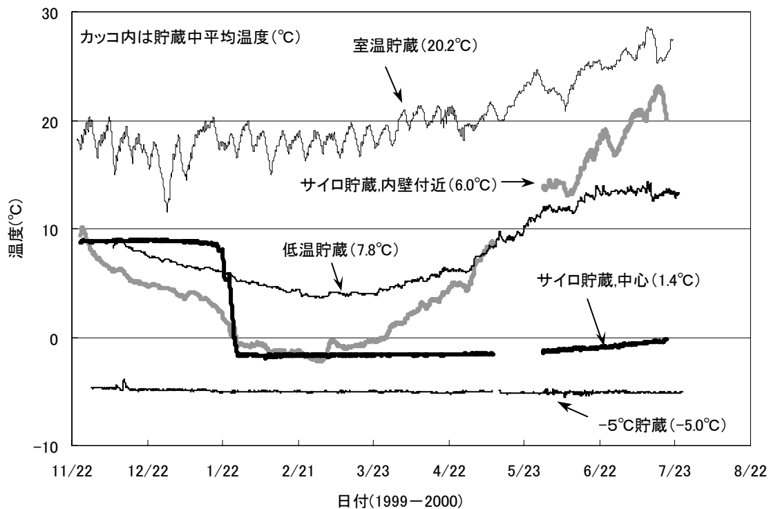
図 46 M10 サイロ貯蔵および対照貯蔵貯の珪温度 (ほしのゆめ)
