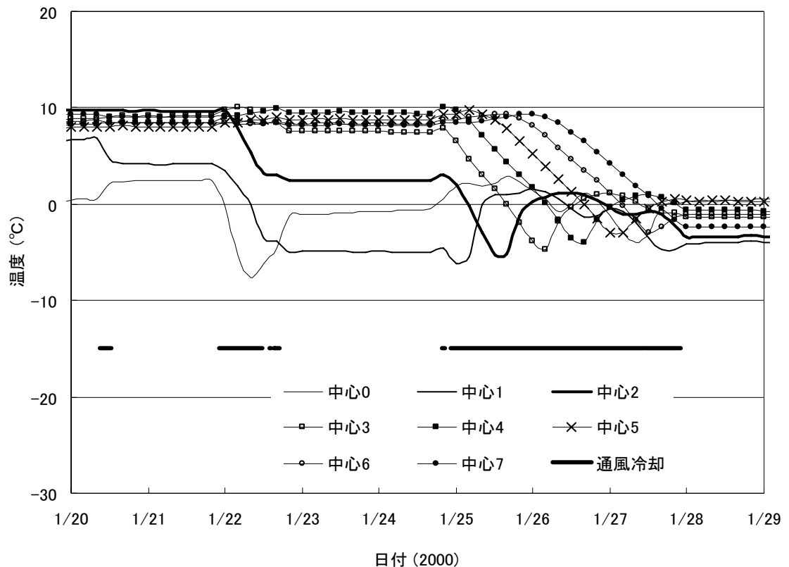
図12 通風冷却時のM10サイロ中心部の籾温度
