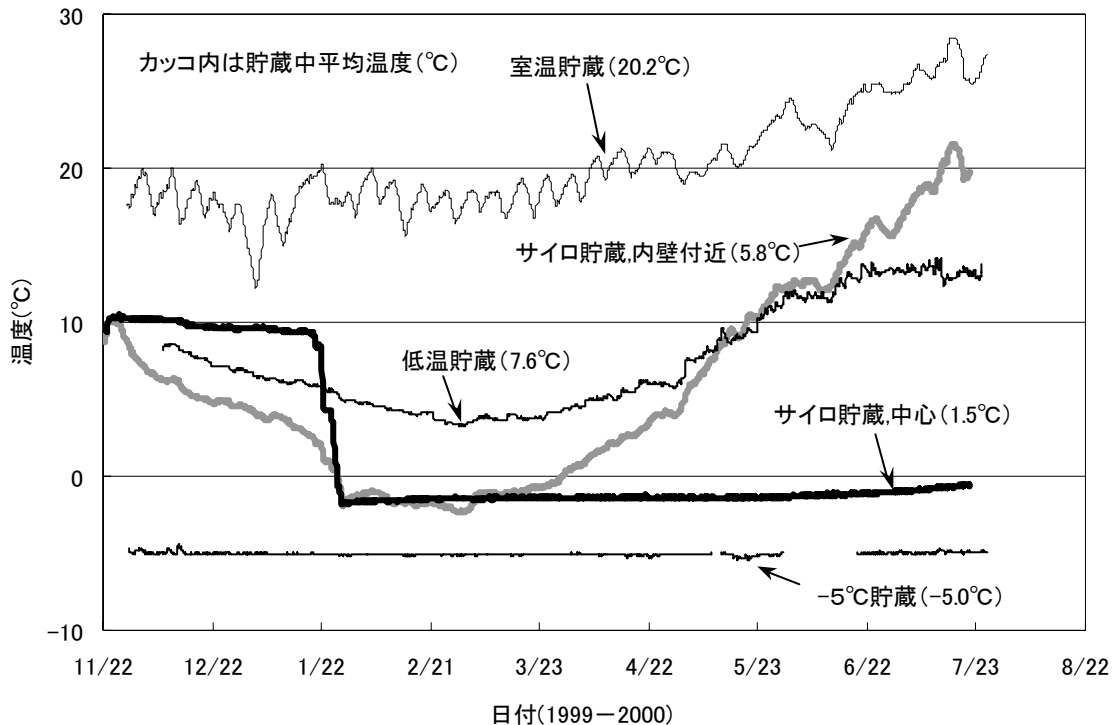
図 45 M9 サイロ貯蔵および対照貯蔵の珪温度 (きらら 397)
