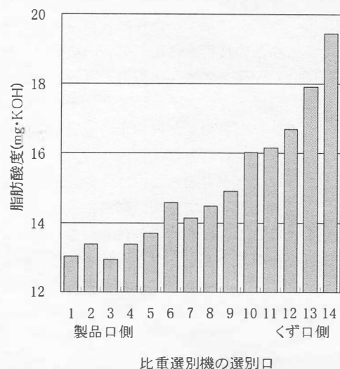
図5 比重選別機の選別口14等分試料の粳摺後玄米の脂肪酸度
