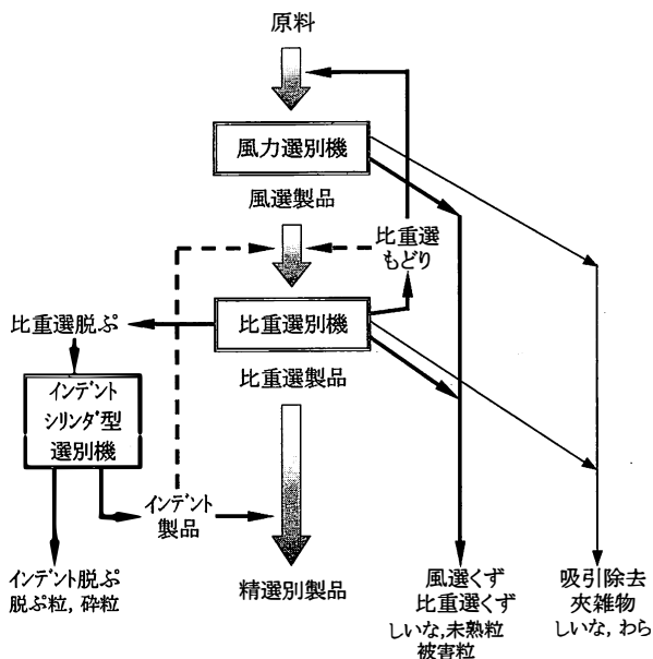
図6 最適な籾精選別システムの流れ図
