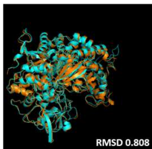
HEME - Fe-S
