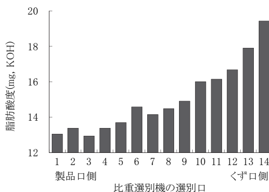
図12 比重選別機の選別口14等分試料の粗摺後玄米の脂肪酸度
