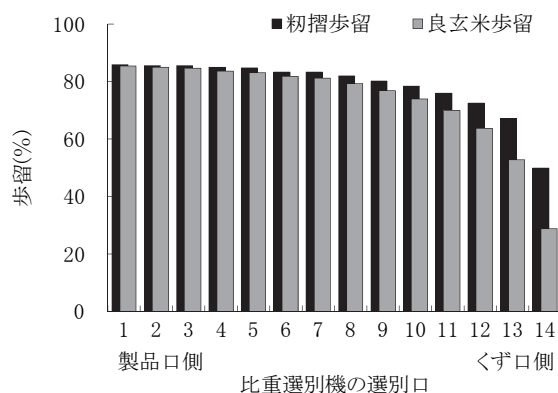
図11 比重選別機の選別口14等分試料の粗摺歩留と良玄米歩留
