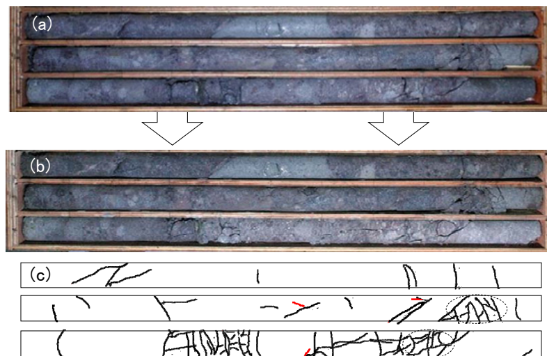
図5 ボーリングコアの状況と亀裂発生を観察例
