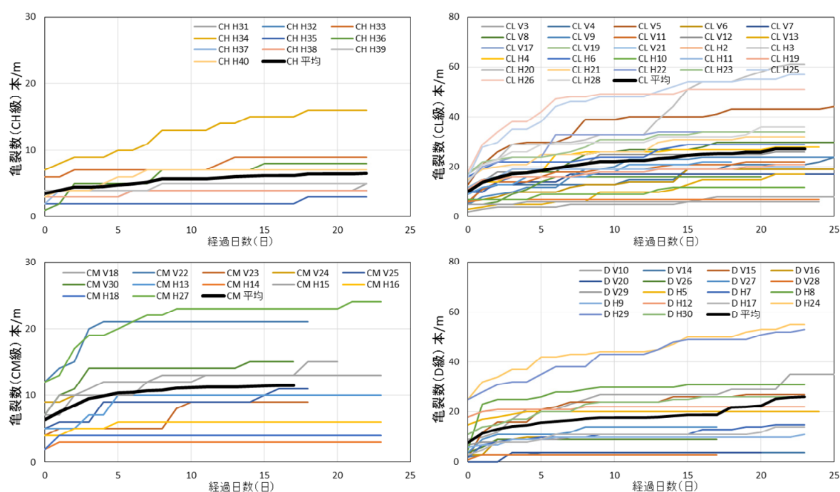
図 7 岩級区分に応じた亀裂数の経時変化
