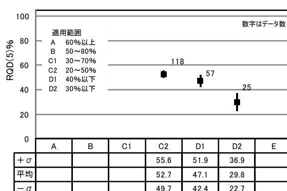
剥離性に富まない古生層～深成岩・火山岩
