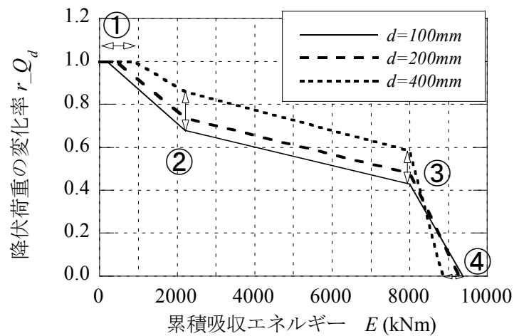
図 3.15 復元力モデルの降伏荷重の変化率と累積吸収エネルギーの関係
