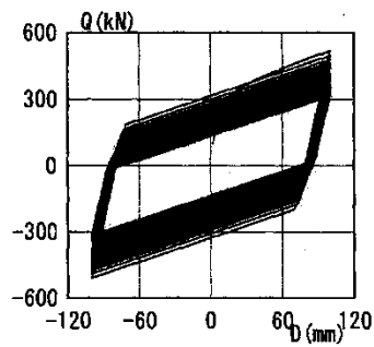
(c) 荷重変形関係 (解析)
