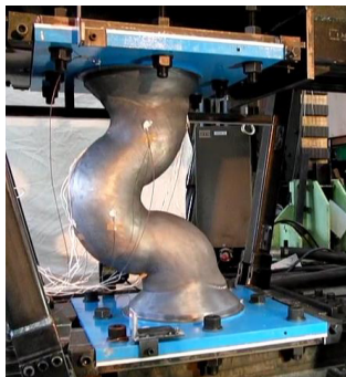
(a) 試験体状況
