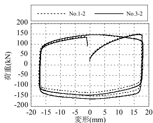
図 5.6 試験体 No. 1 および No. 3 の荷重変形関係 (加力ケース 2)
