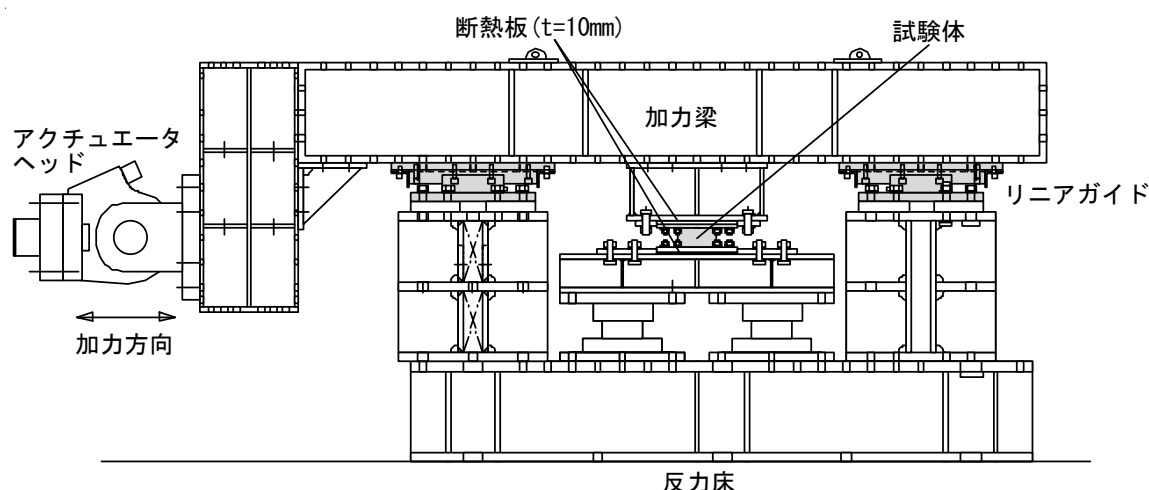
図 5.2 試験装置
