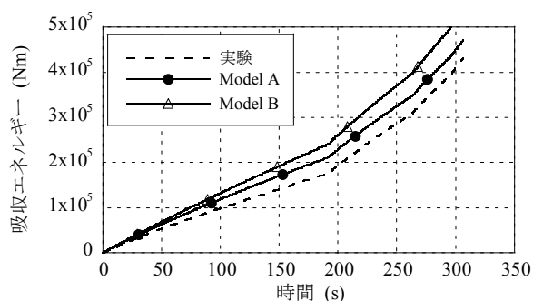
図 5.33 漸増連続正弦波加力の吸収エネルギー
