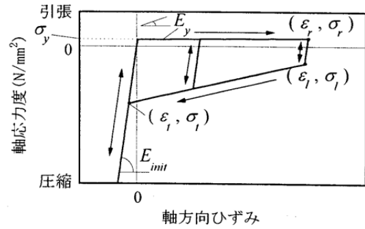
図 1.41 並列軸ばねの復元力特性 43)
