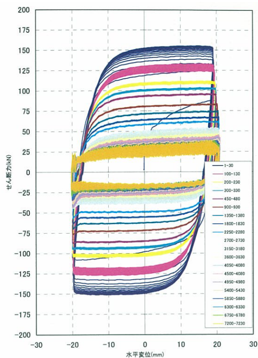
(d) 加振振動数 0.33Hz、振幅 \pm 20\text{mm} 16)
