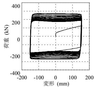
(b) 重力考慮
