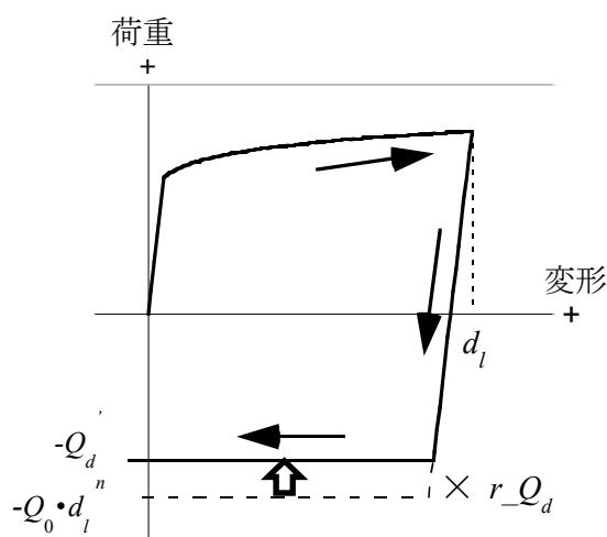
図 3.16 復元力モデルにおける繰返し変形による降伏荷重の変化
