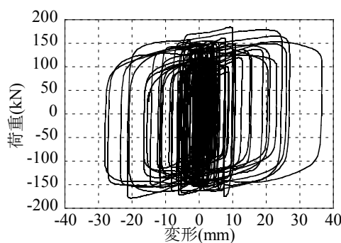
図 5.13 地震応答波加力の荷重変形関係
