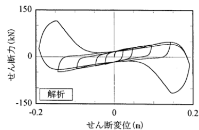
図 1.42 並列軸ばねモデルによる水平荷重変形関係 43)
