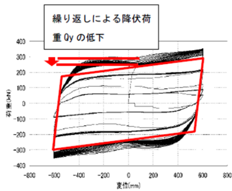
図 4.4 鋼材ダンパーの繰返し変形実験結果 3)
