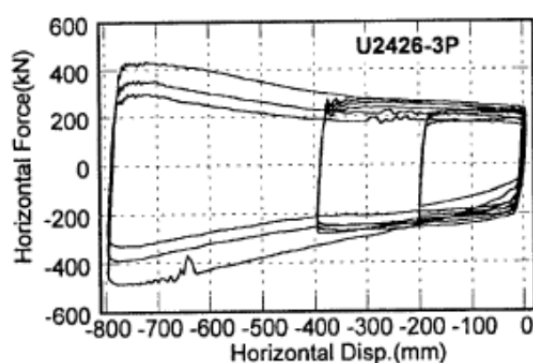
(b) 加振振動数 0.33Hz、800mm 片振り加振 15)
