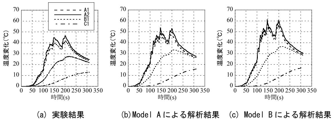
図 5.41 地震応答波加力の温度変化
