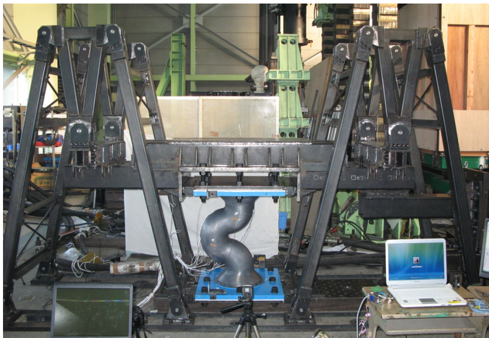
写真 3.1 試験状況
