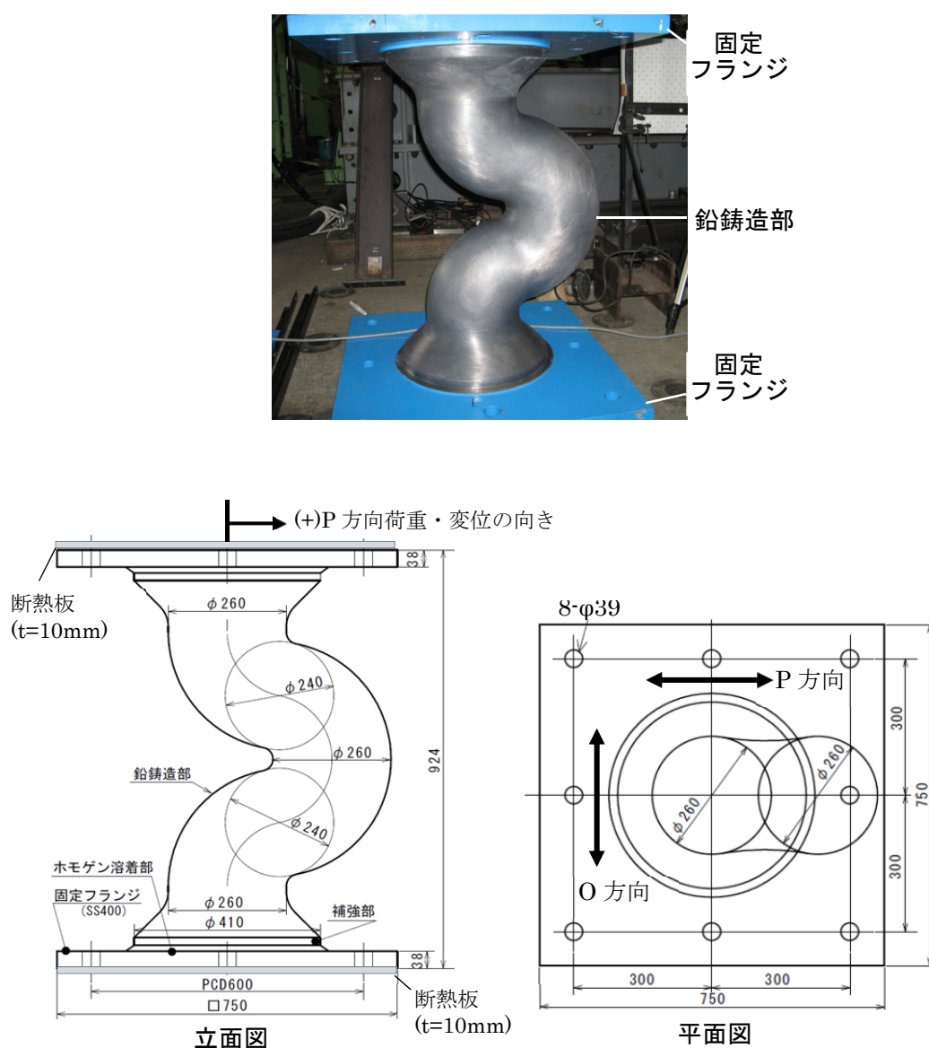
図 3.1 試験体
