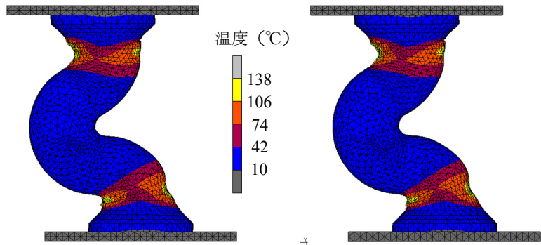
(b) 重力非考慮時温度分布
