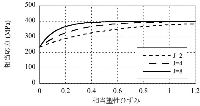
図 5.20 Chaboche モデルの応力ひずみ曲線
