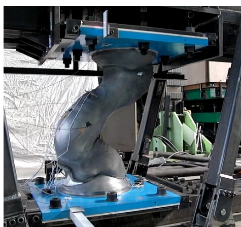
(c) \pm 200\text{mm} 30 サイクル目
