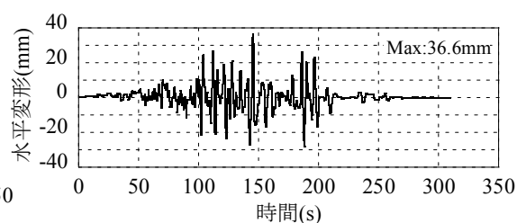
図 5.4 地震応答波加振（試験体 No. 3）
