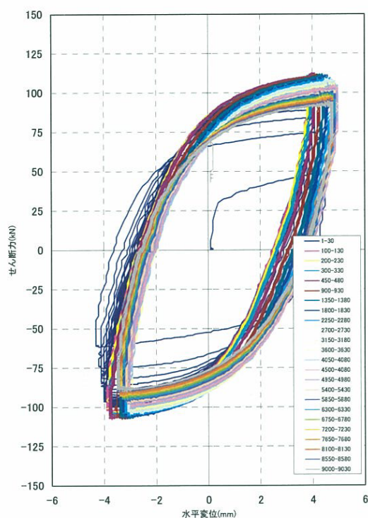
(c) 加振振動数 0.33Hz、振幅 \pm 5\text{mm} 16)
