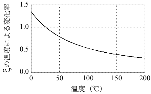
図 5.23 \xi の温度依存性
