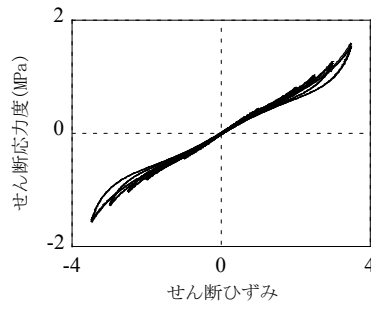
(a) 実験結果
