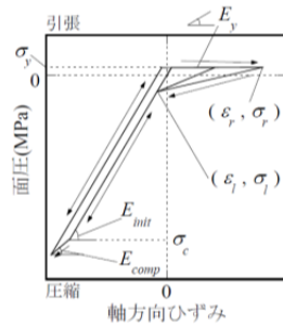
図 2.20 並列軸ばね特性
