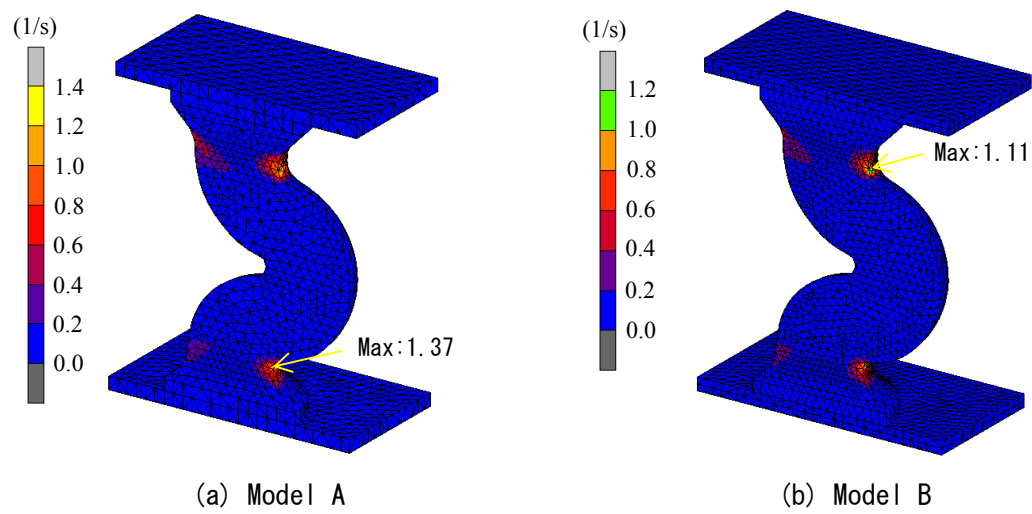
図 5.59 解析 6 秒時の相当塑性ひずみ速度
