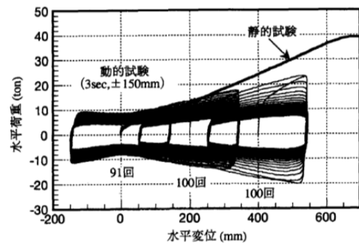
図 1.8 U180 型ダンパーO 方向荷重変形関係 7)
