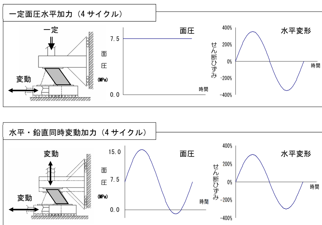
図 2.2 加力方法
