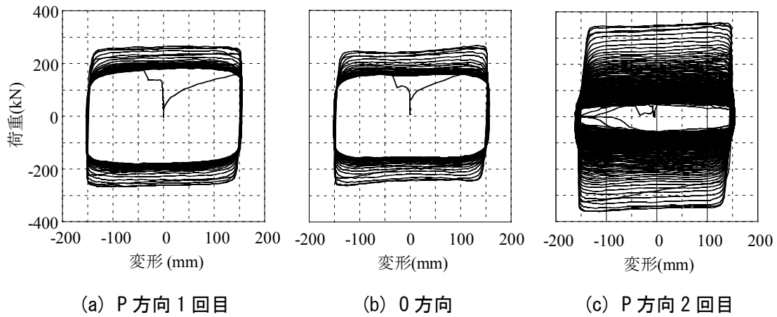
図 3.8 試験体 No. 2 荷重変形関係
