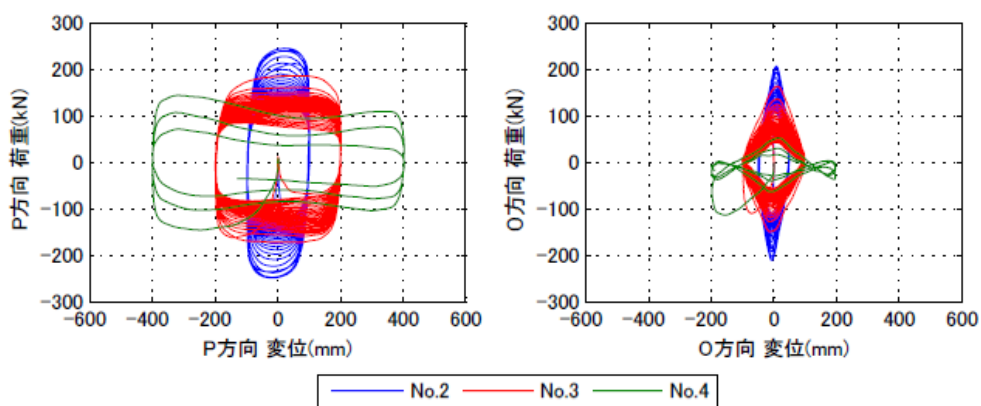
図 1.21 連続楕円正弦波加振 荷重変形関係 17)
