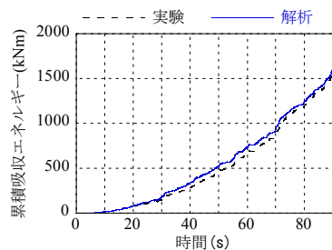
図 5.77 長周期地震動応答波加力
