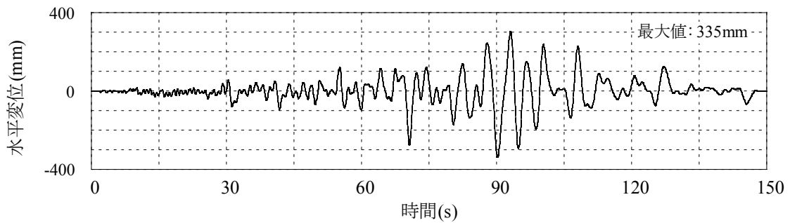
(b) 地震応答波加振
