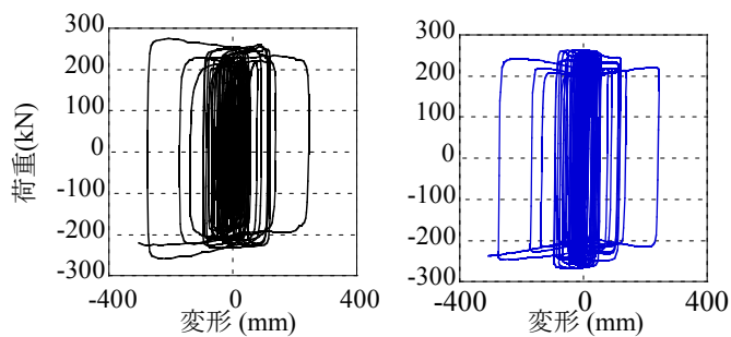
(a) 実験結果
