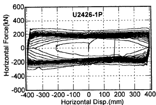
(a) 加振振動数 0.33Hz、振幅 \pm 400\text{mm} 15)
