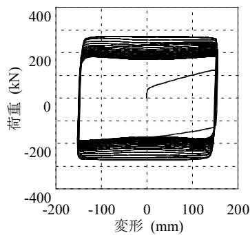
(a) 重力非考慮
