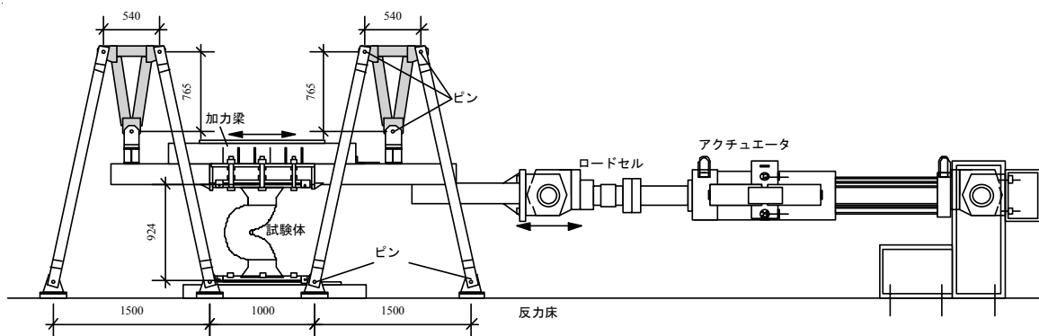
図 3.2 試験装置
