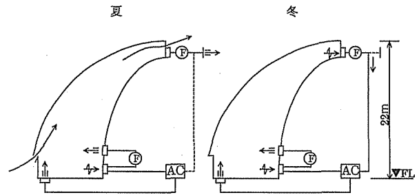
図-6 イントランスホール空調システム概念図
