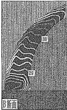
図-4 イントランスホール 断面温度分布
