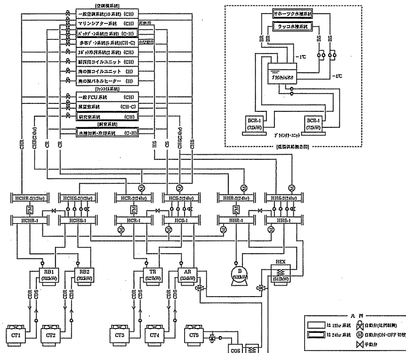
図-3 熱源供給系統概念図
