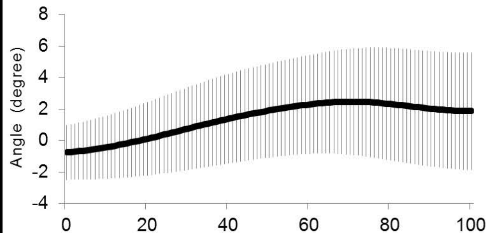
Knee ADD(+)/ABD(-)
