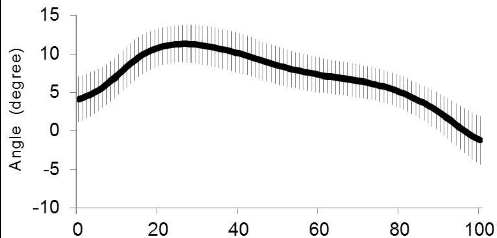
Hip ADD(+)/ABD(-)
