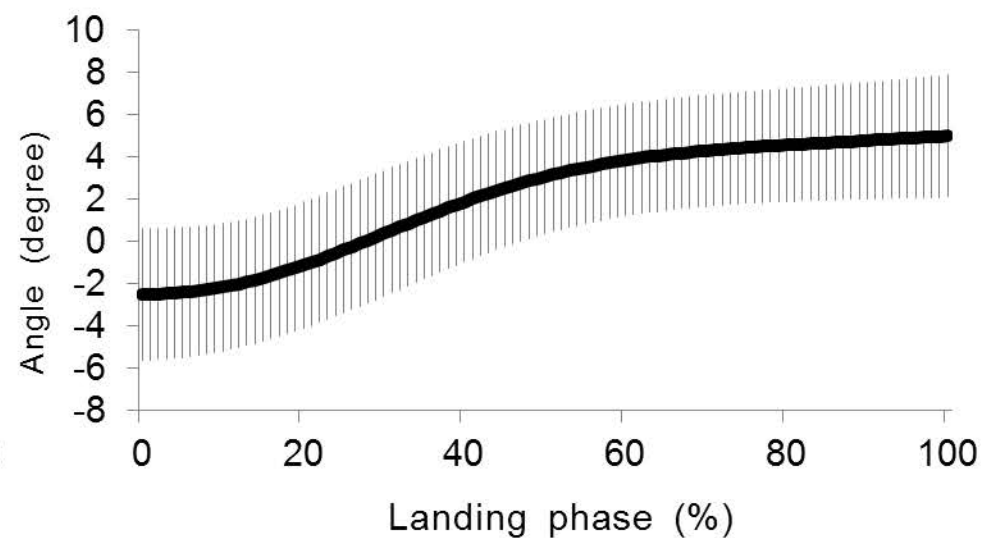
Rearfoot ER(+)/IR(-)
