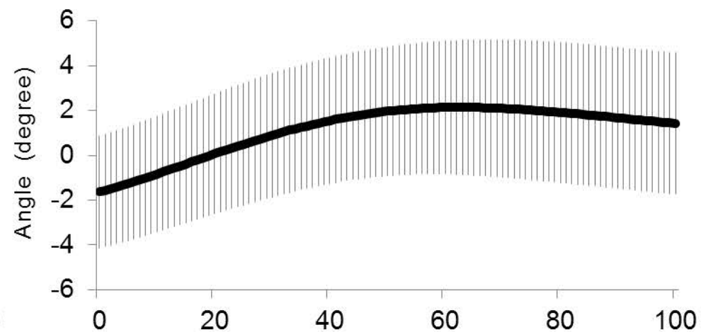
Knee IR(+)/ER(-)
