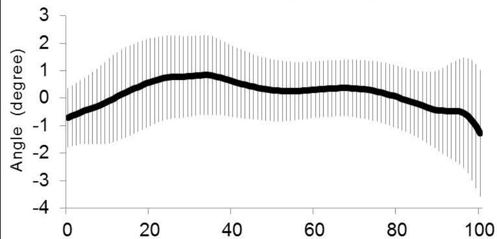
Knee ADD(+)/ABD(-)
