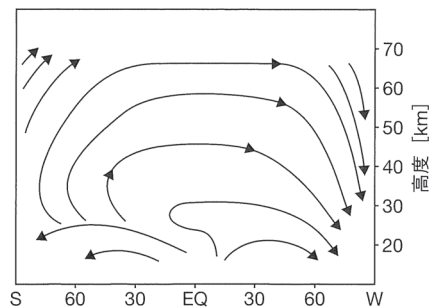
図 ブリュウワードブソン循環の概念図を流線で示したもの 1) 。縦軸は高度、横軸中央のEQは赤道、左端のSは夏極、右端のWは冬極を示す。
