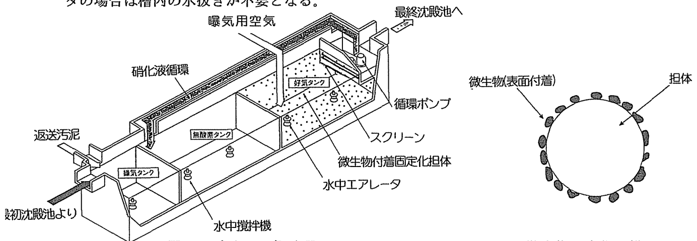
図1 反応タンク概略図
