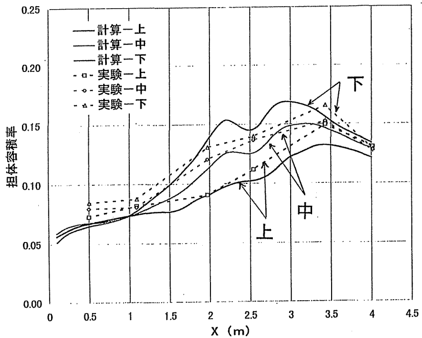
図 3.3 担体容積率分布の実験結果と計算結果の比較(実験槽全面曝気式)
