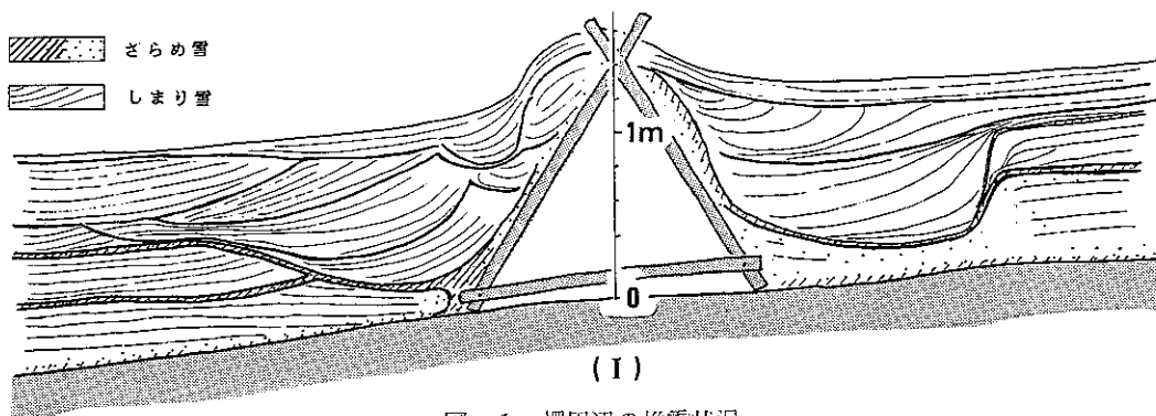
図-1 柵周辺の堆雪状況
