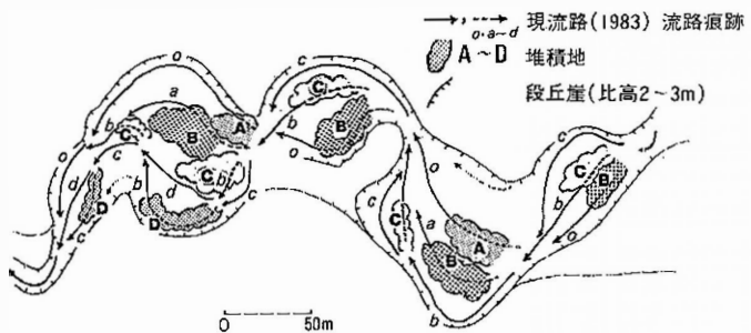
図-3 アユマナイの土砂移動状況
