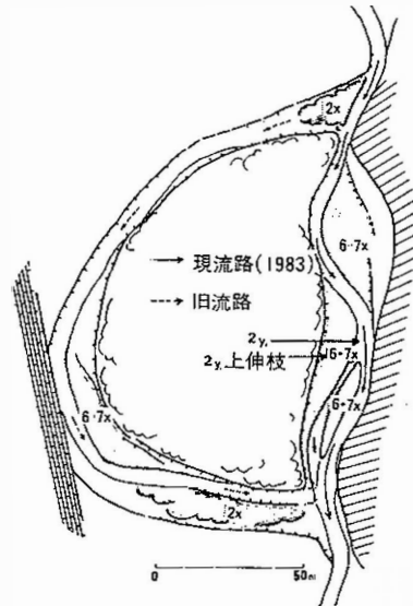
図-2 流路変動・旧流路への再流入(1983現在)
