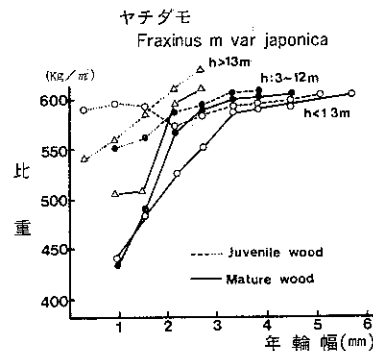
図-2 ヤチダモ材比重の生長効果
