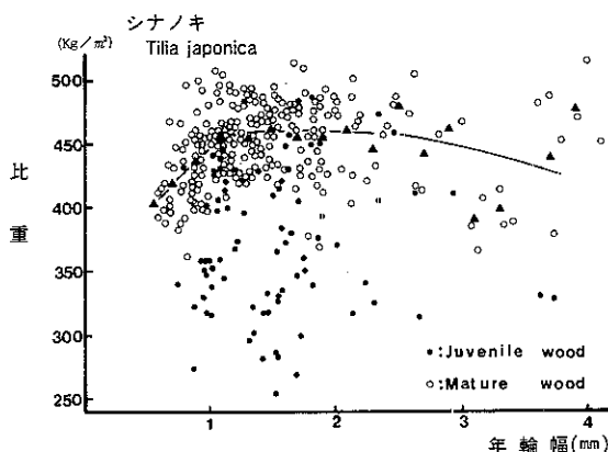
図一 4 シナノキ材比重の生長効果
