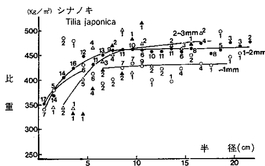
図一 3 シナノキ材比重の年齢効果
