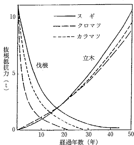
図一3 伐根ならびに植栽後の経過年数と抜根抵抗 (全国林業改良普及協会編：林業技術ハンドブックより引用)
